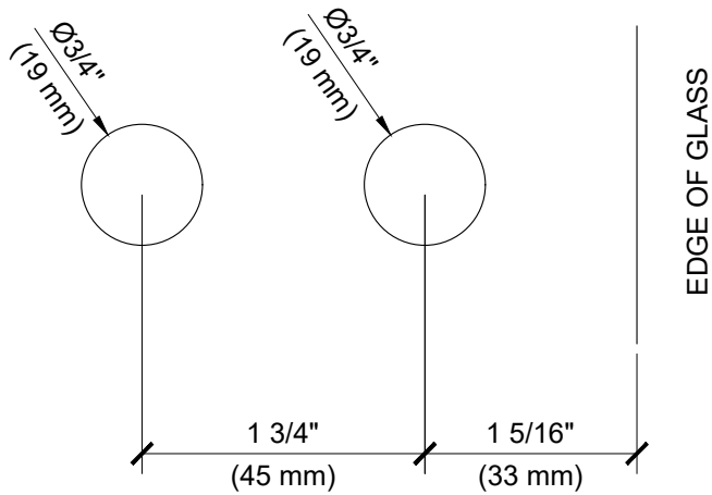
3 FHDxx HINGE N.T.S. ARCH. REF.:
