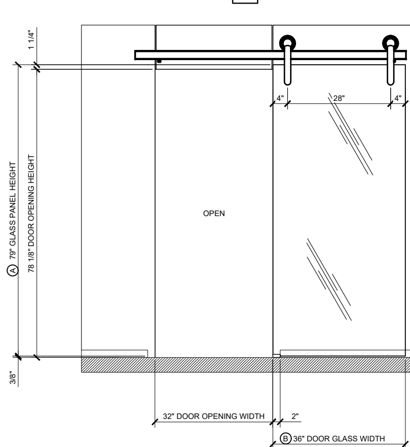
2B ELEVATION
