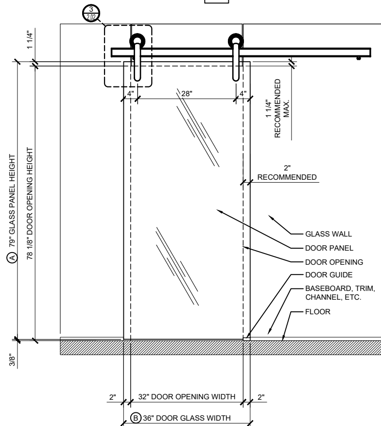
1B ELEVATION
