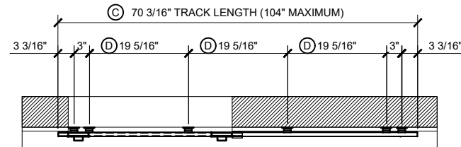
1A PLAN
