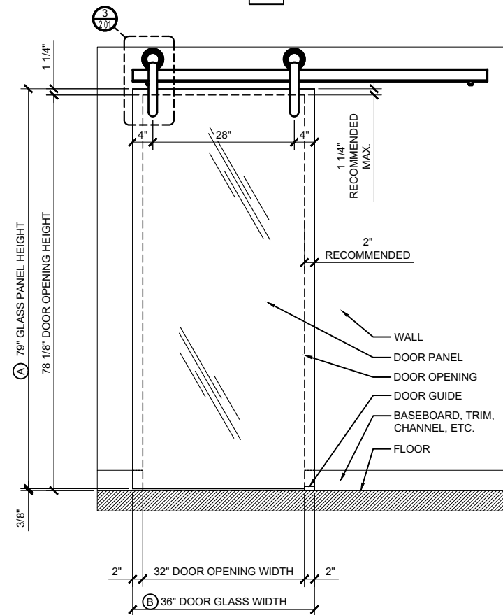
1B ELEVATION
