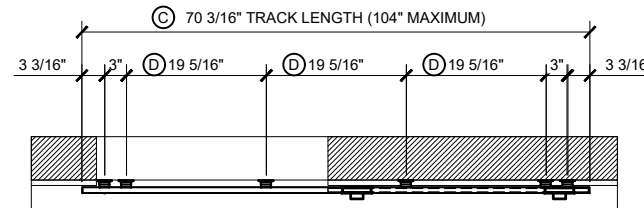
2A PLAN
