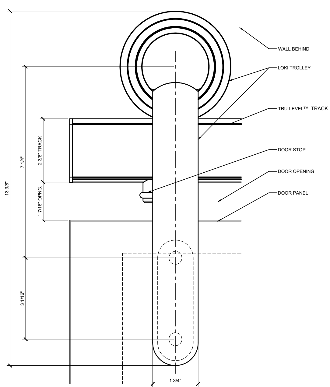
3 DOOR SLIDER ELEVATION
