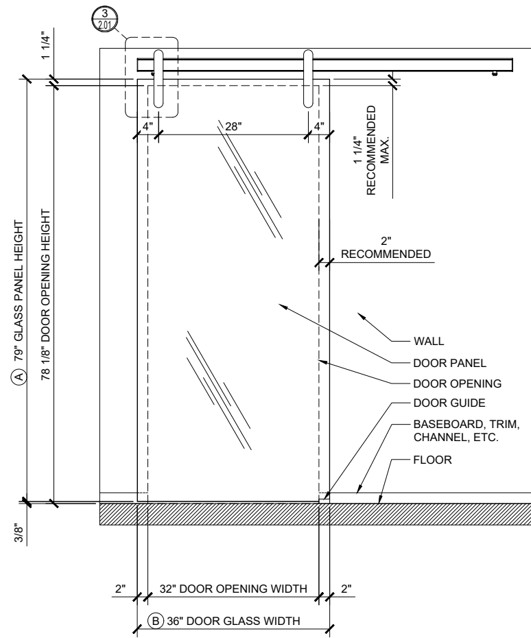
1B ELEVATION
