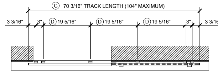
2A PLAN
