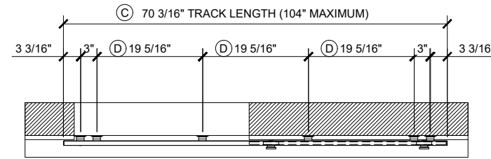
2A PLAN
