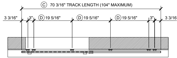
1A PLAN
