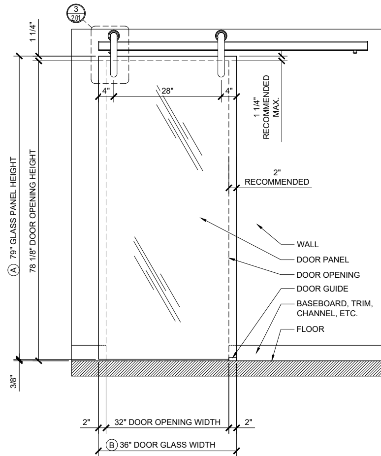
1B ELEVATION
