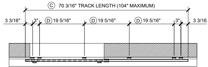
1A PLAN
