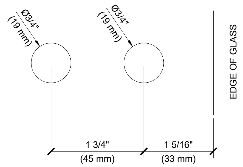
2 FHSxx HINGE N.T.S.
