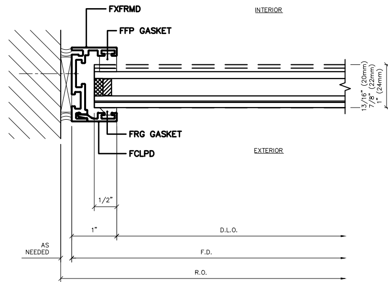
① JAMB DETAIL @ FRAME XL 20-24.76 1'-0\"/>
