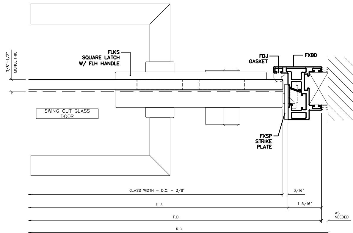
④ DOOR JAMB DETAIL @ LOCK 1'-0\"/>
