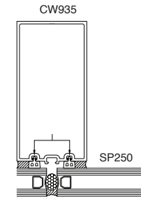
③ JAMB
