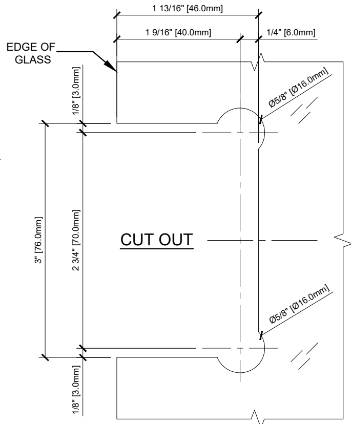
SWING DOOR GLASS
