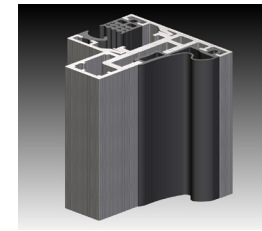
Door Jamb/Header at Sidelite/Transom
