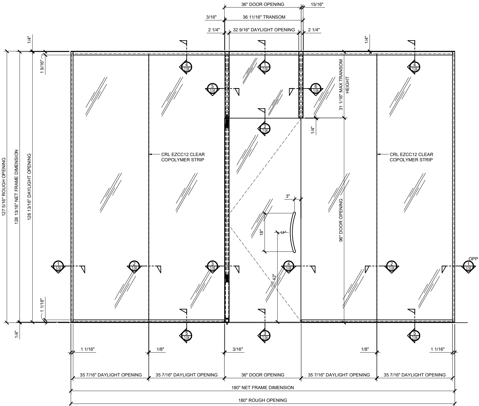
② ELEVATION
