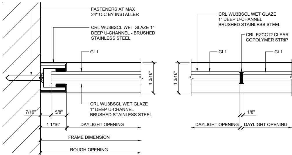
① WALL JAMB DETAIL
