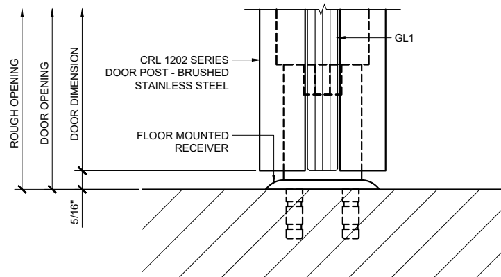
③ DOOR SILL DETAIL
