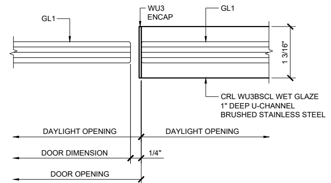
④ DOOR JAMB AT SIDELITE
