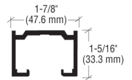
STANDARD D7 OVERHEAD TRACK SPECIFY D1018 ASSEMBLY
