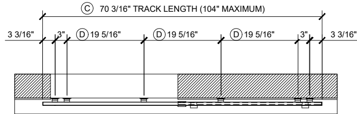
2A PLAN
