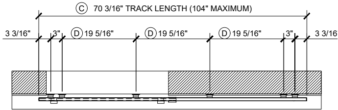
1A PLAN
