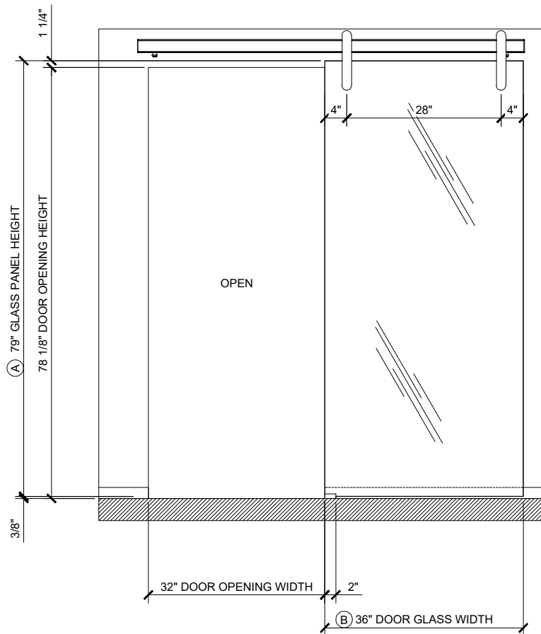
2B ELEVATION
