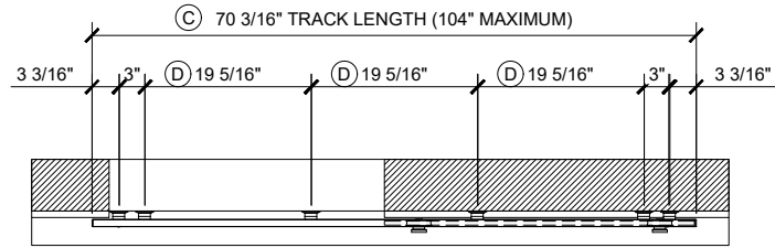
2A PLAN
