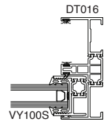
7 FIXED JAMB
