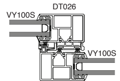
6 INTERLOCK
