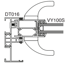
5 OPERABLE JAMB
