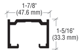
STANDARD D7 OVERHEAD TRACK SPECIFY D1025 ASSEMBLY
