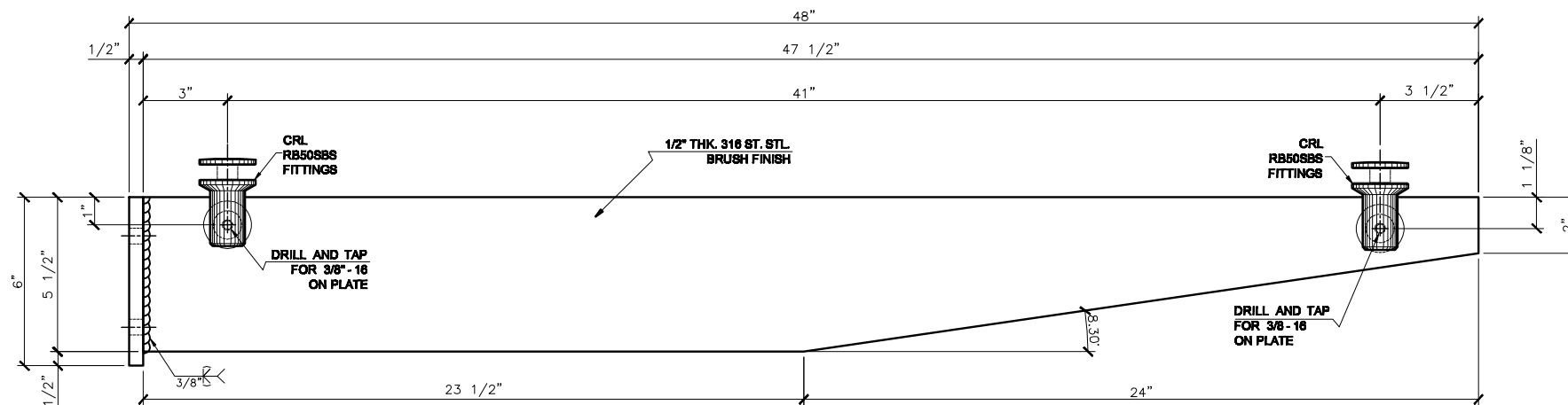
○ CRL 48" - GAB48 Scale: 1 = 6
