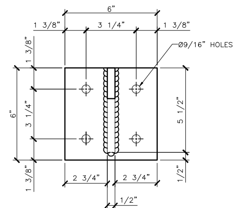
○ BASE PLATE Scale: 1 = 6
