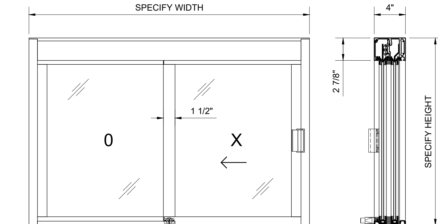
ELEVATION
