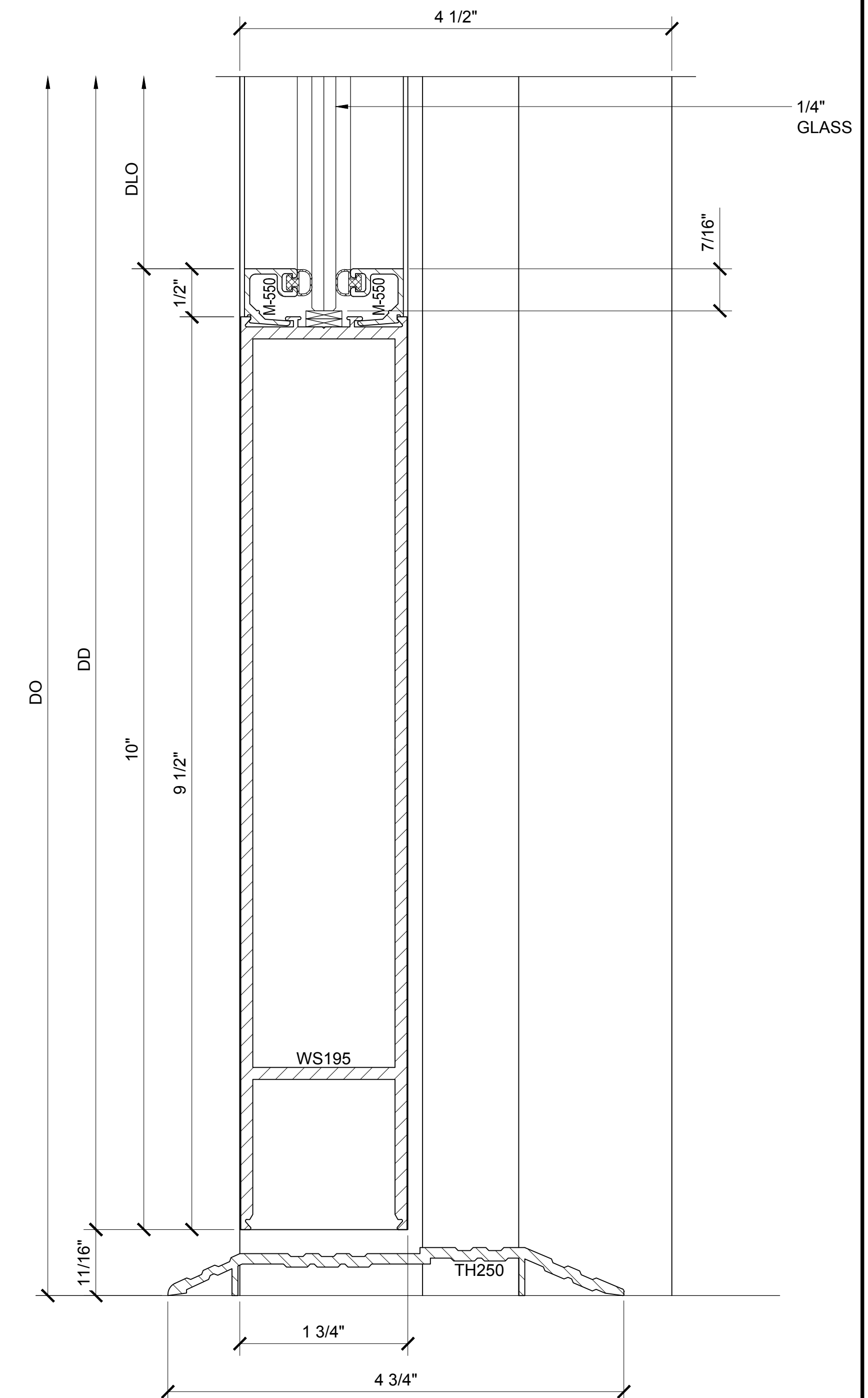
SECTION DETAIL @ ADA DOOR SILL 16
