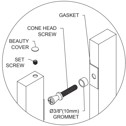
DETAIL A-A
