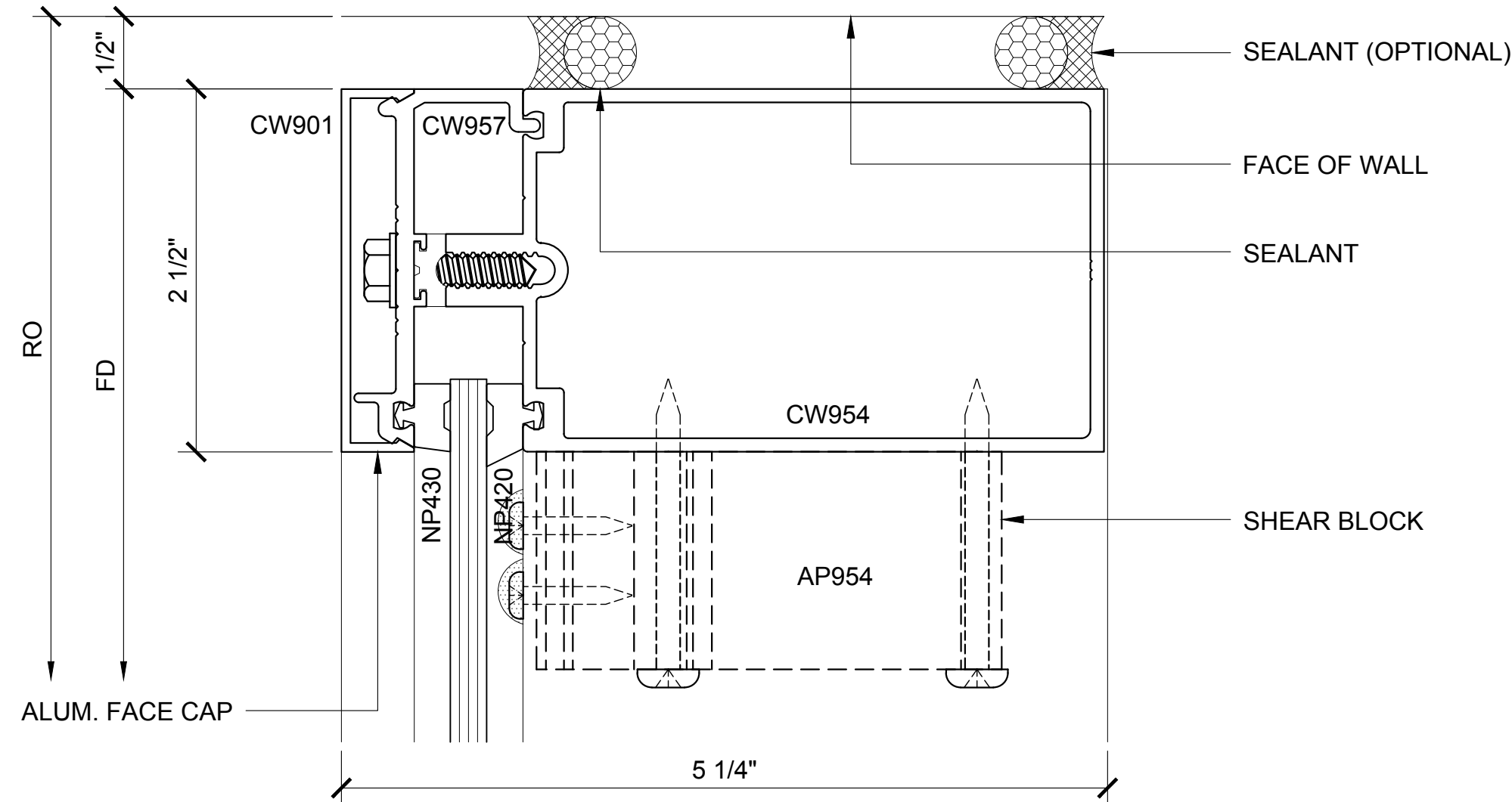
JAMB PLAN 1
