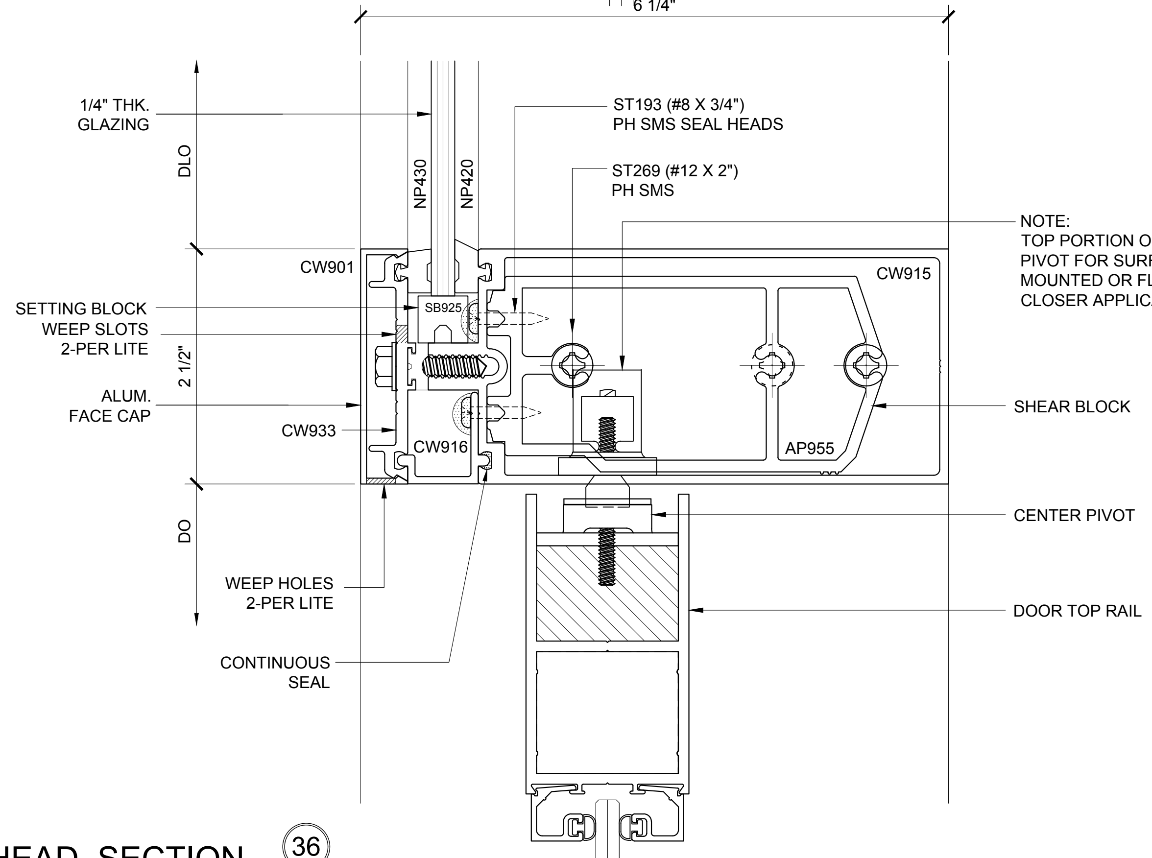
DOOR HEAD SECTION 36
