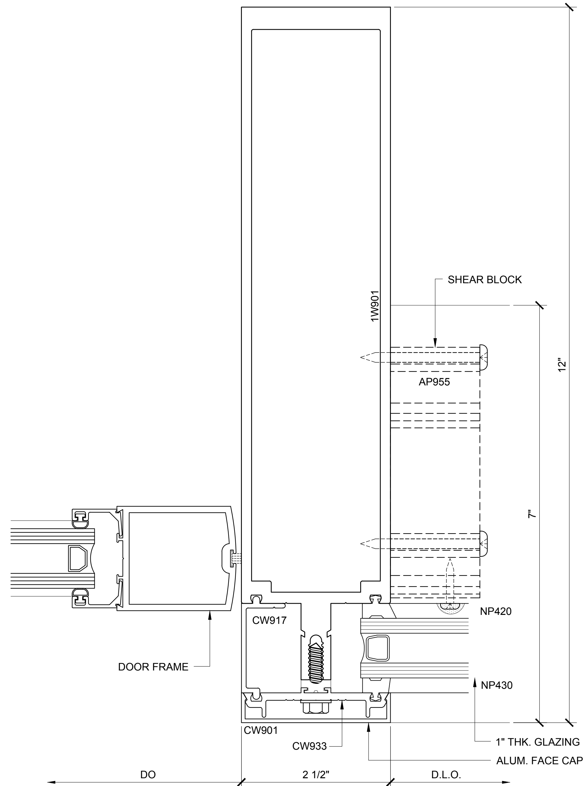
INT. VERT. PLAN (152)
