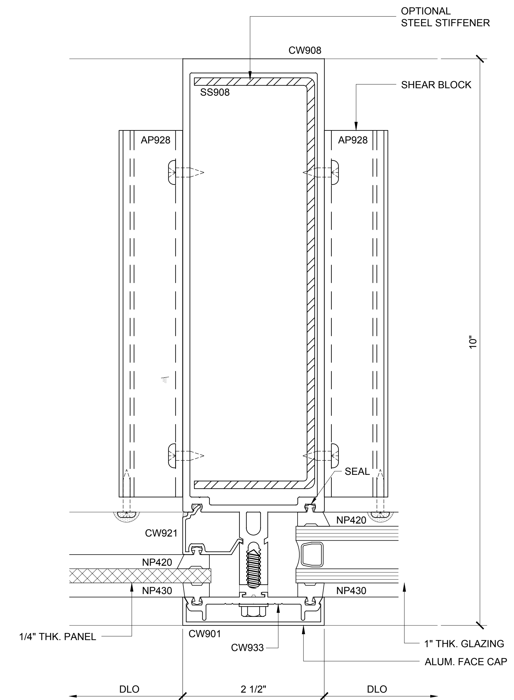
INT. VERT. PLAN 112
