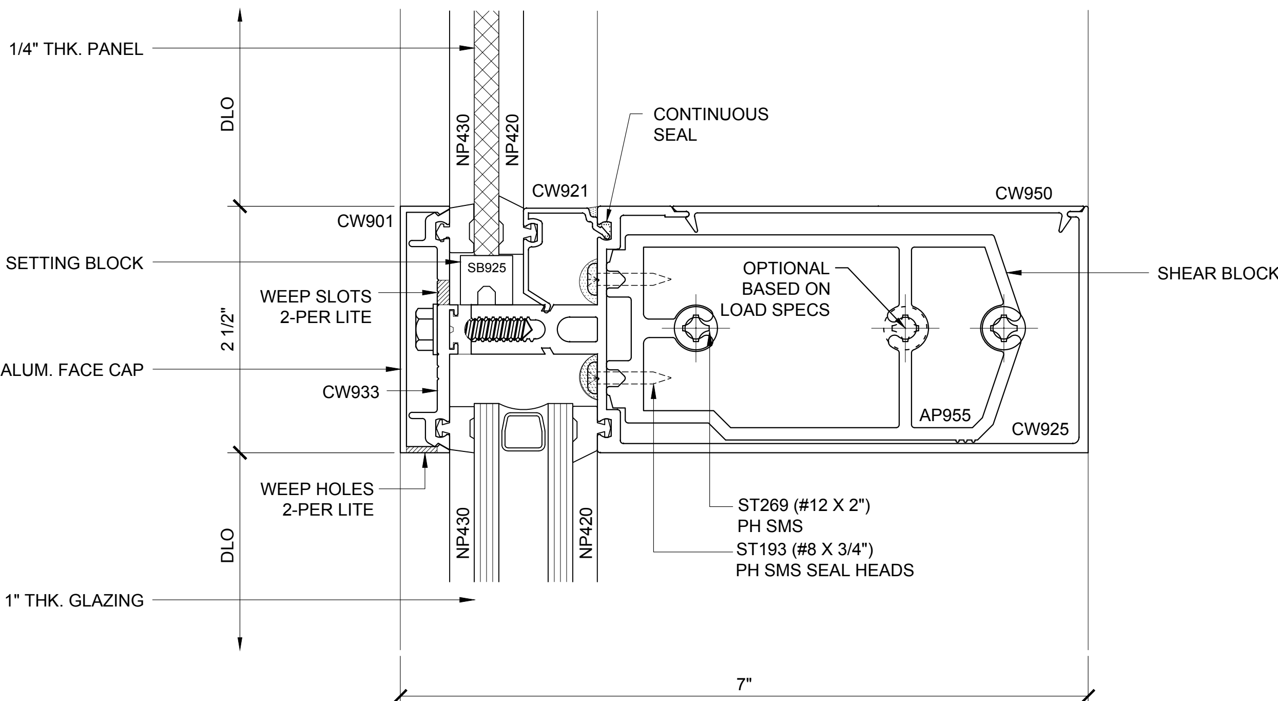
INT. HORIZ. SECTION 107A
