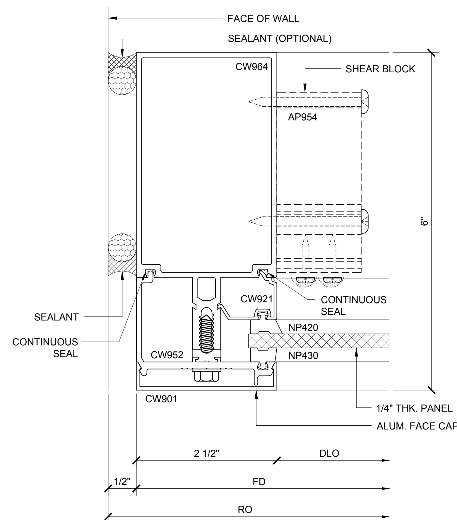
JAMB PLAN 47A
