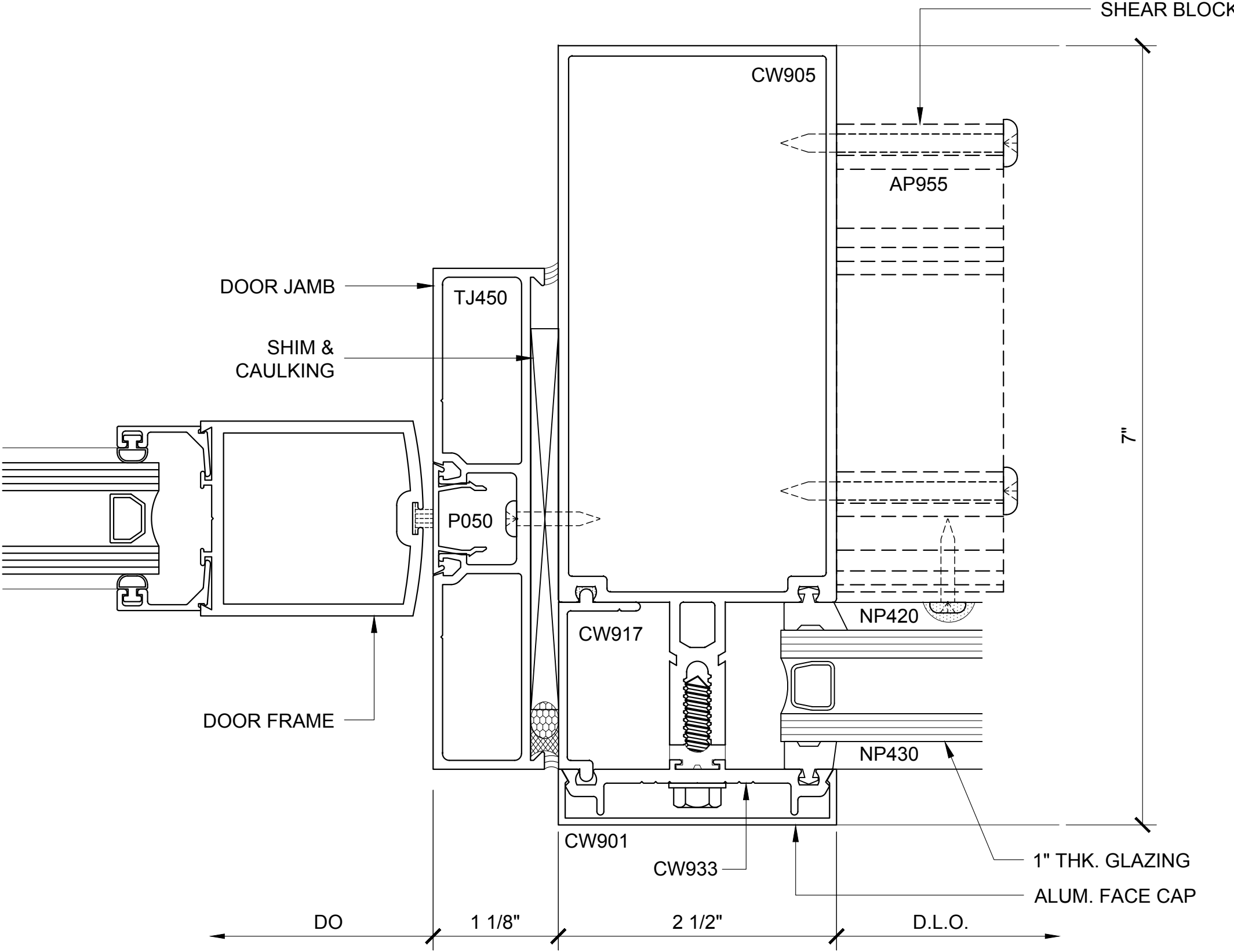
DOOR JAMB PLAN 85
