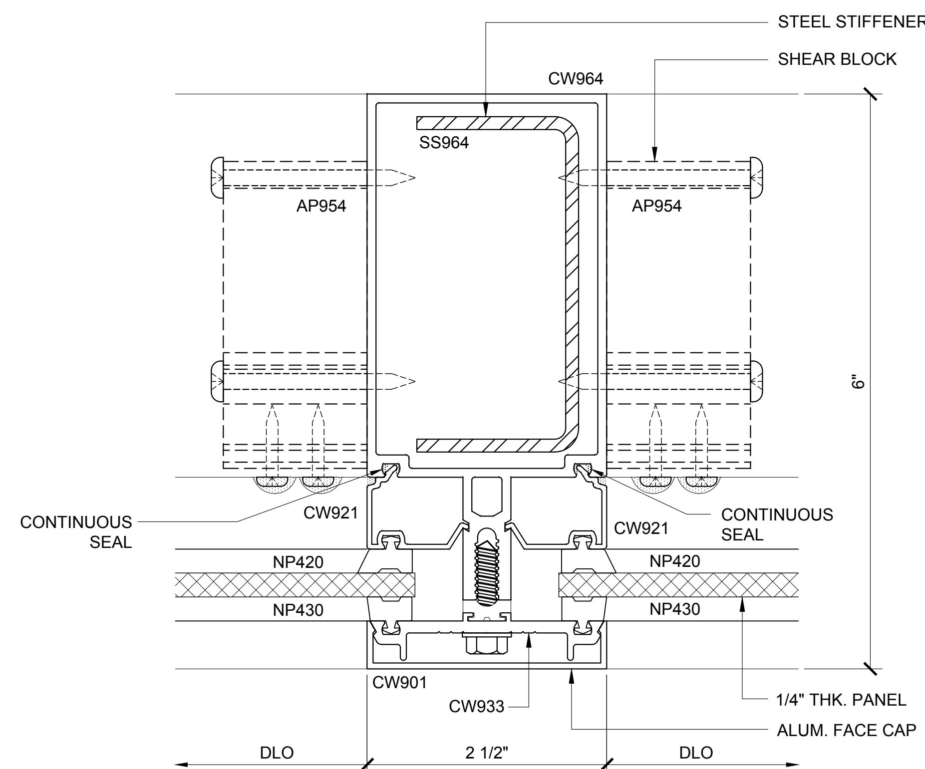
INT. VERT. PLAN (77)
