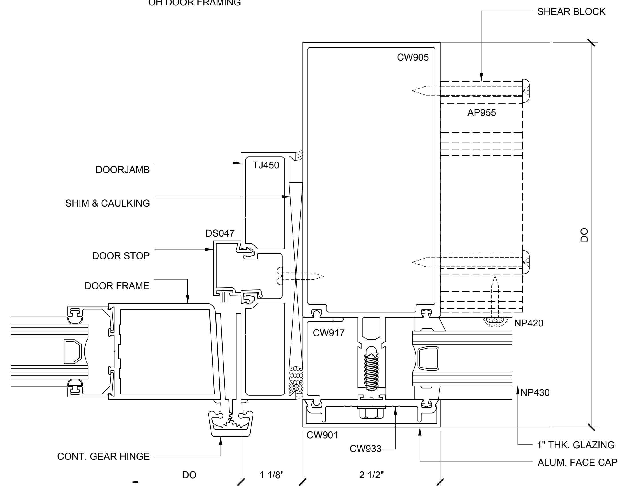
DOOR JAMB PLAN (97)
