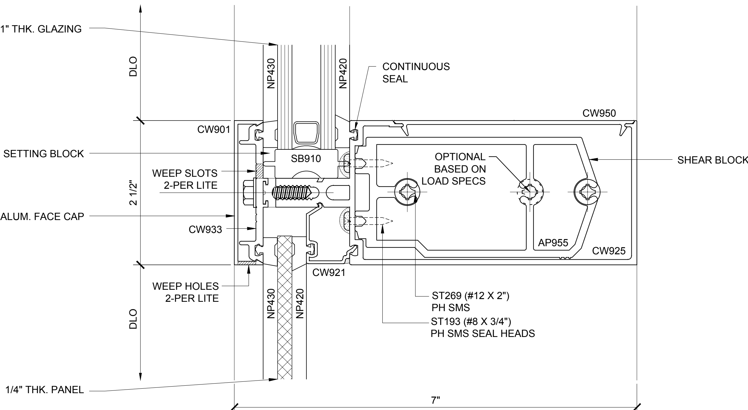
INT. HORIZ. SECTION 107
