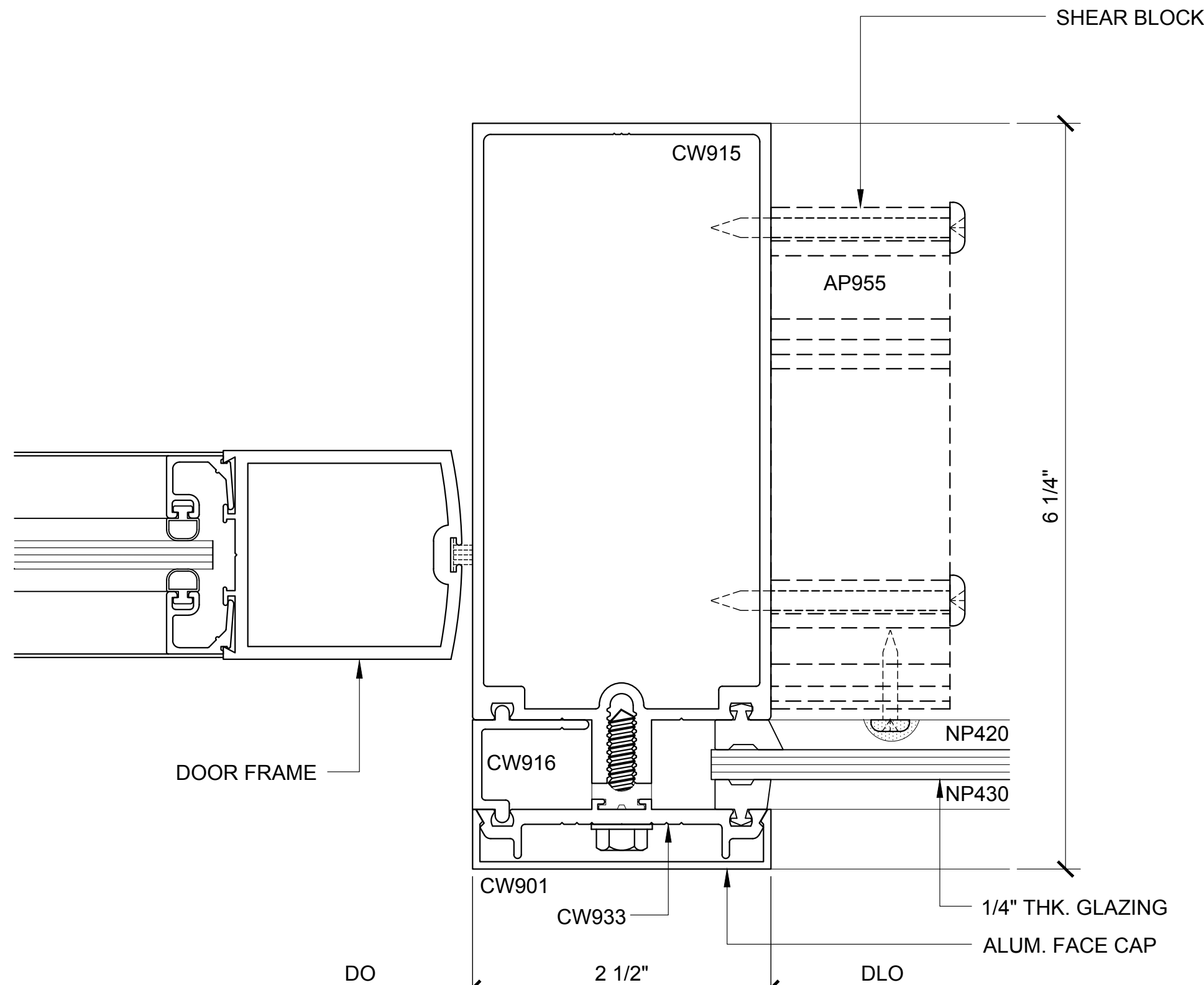
DOOR JAMB PLAN (30)
