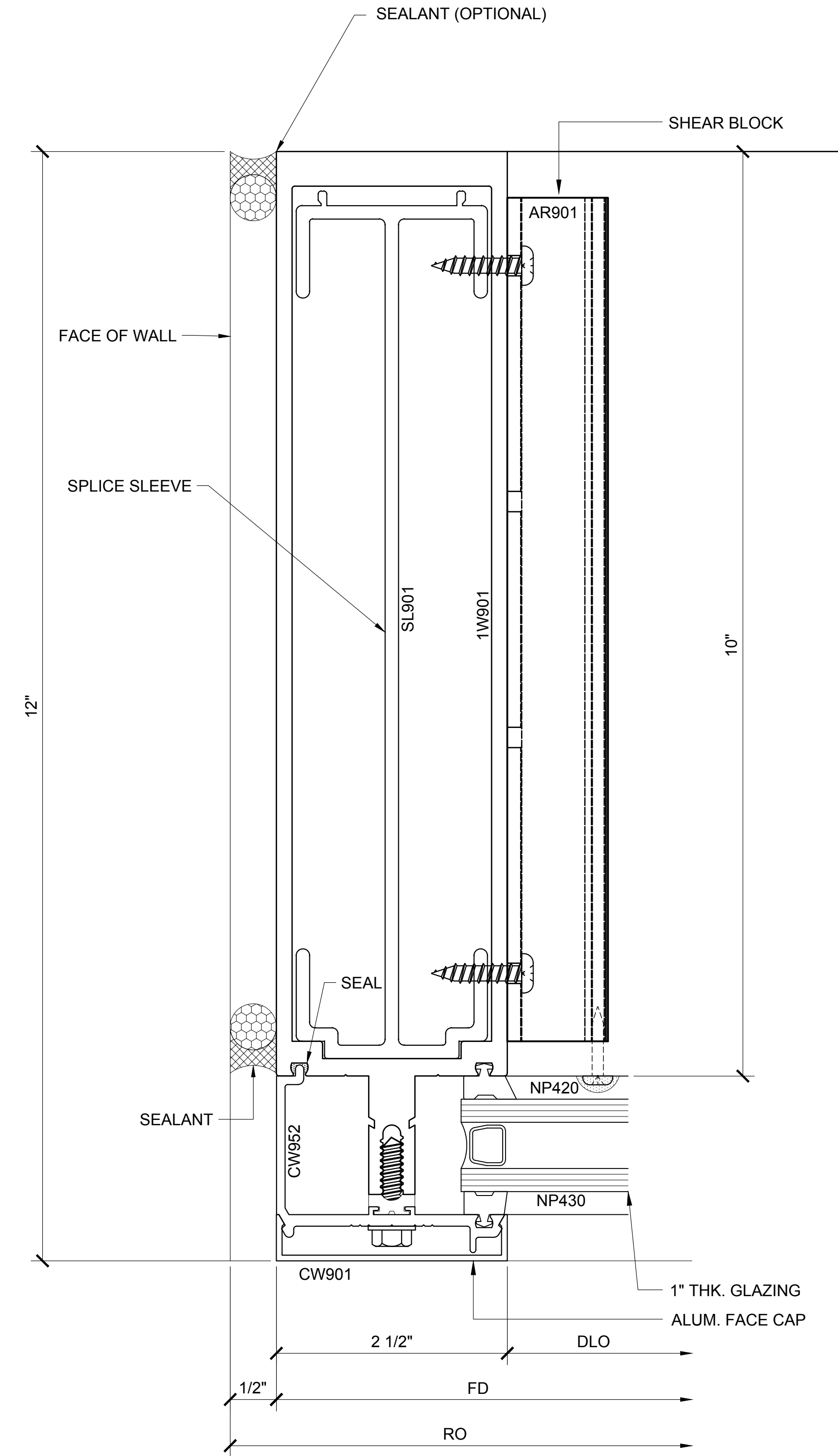
JAMB PLAN 179
