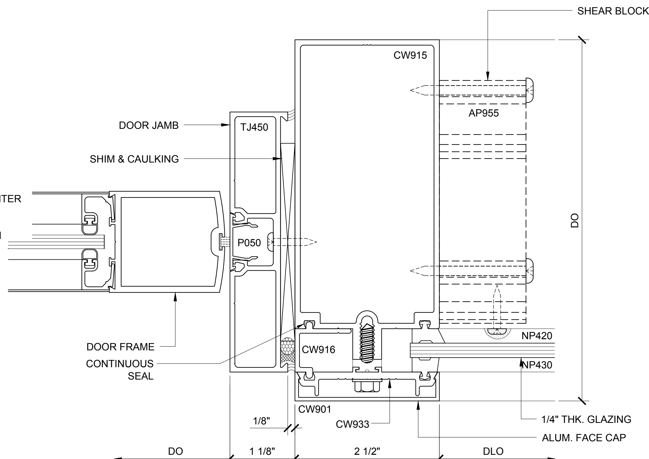
INT. VERT. PLAN (27)
