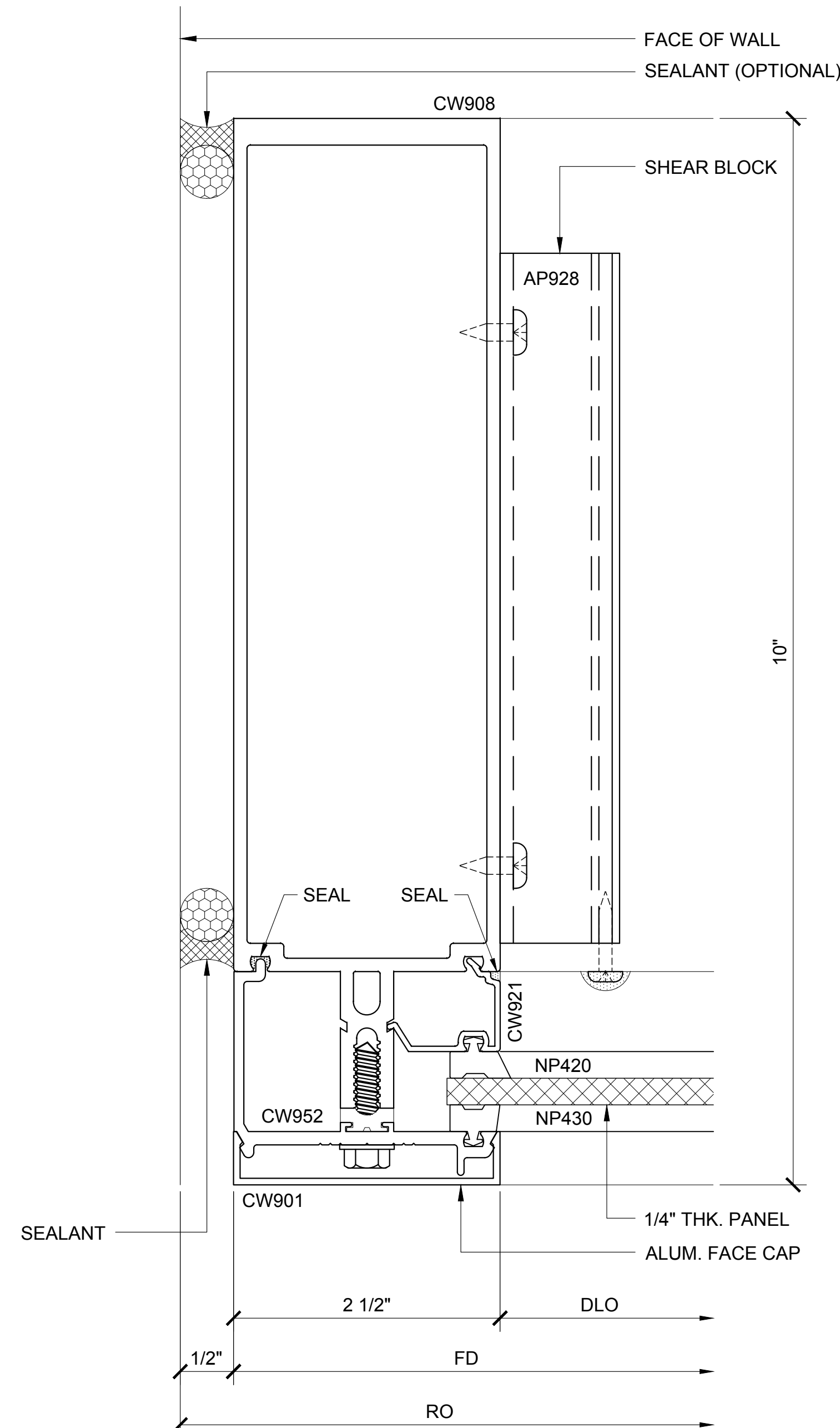
JAMB PLAN 54A
