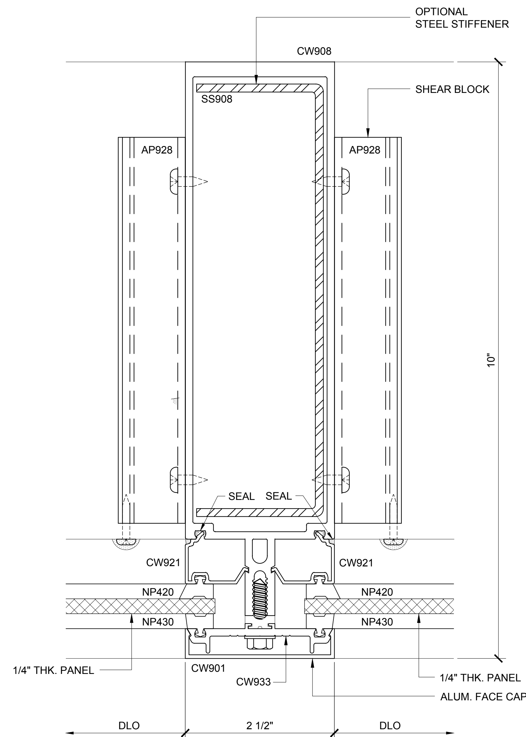
INT. VERT. PLAN 114
