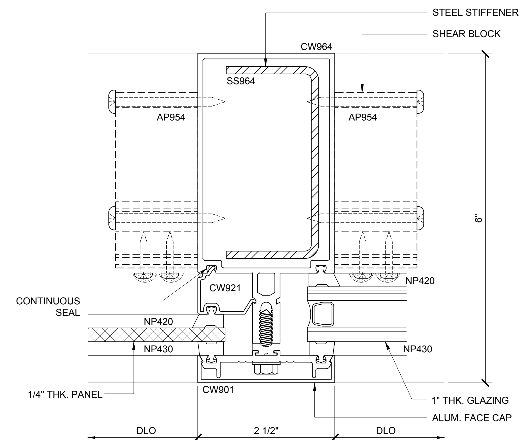
INT. VERT. PLAN (75)
