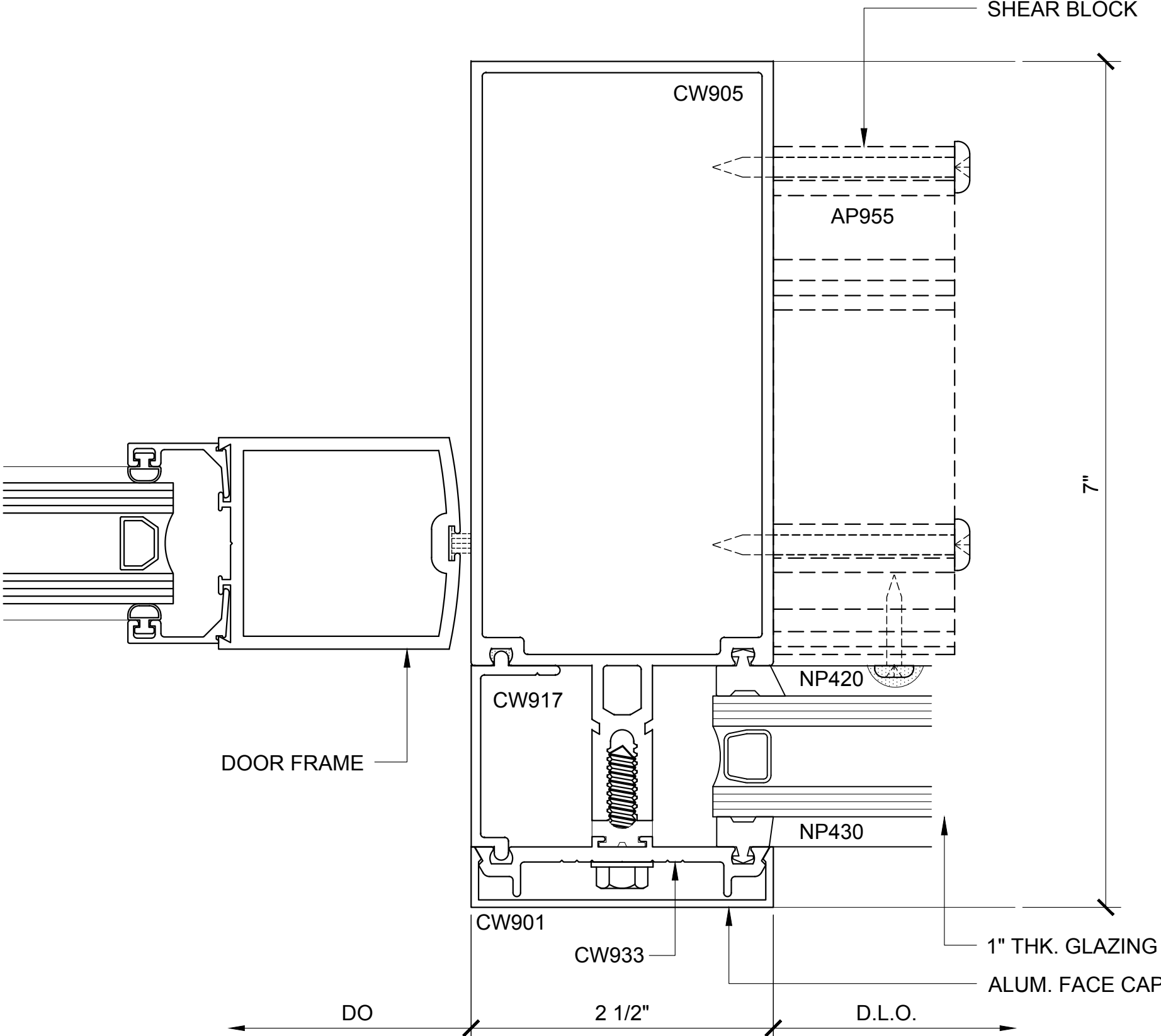
INT. VERT. PLAN 82
