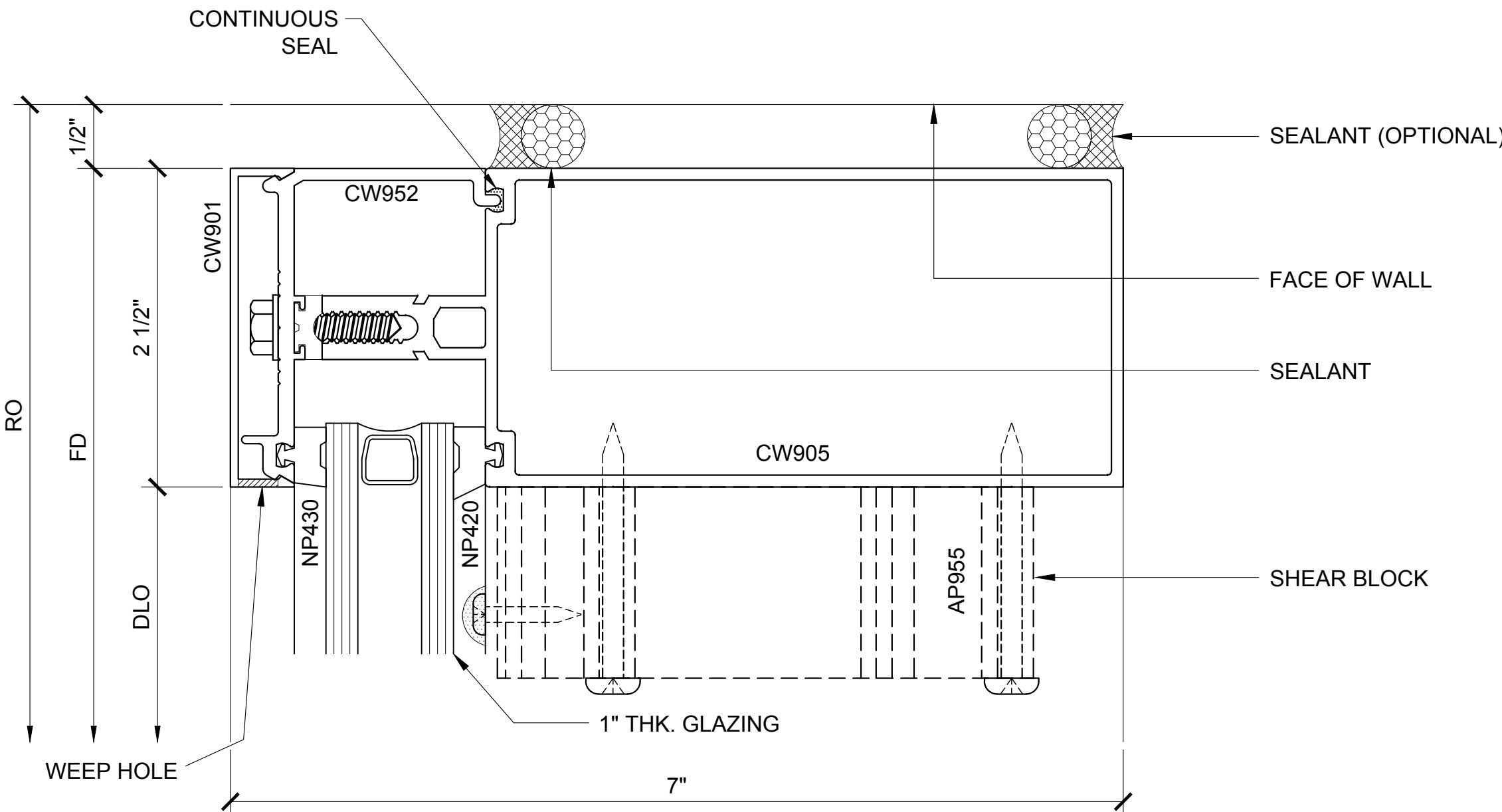
JAMB PLAN 52
