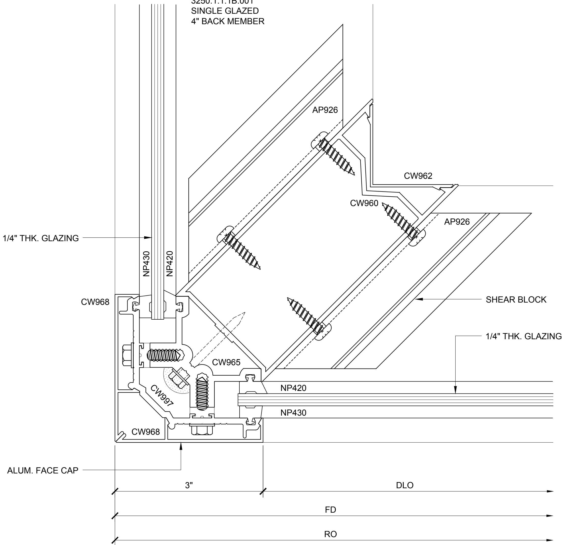
JAMB PLAN 1
