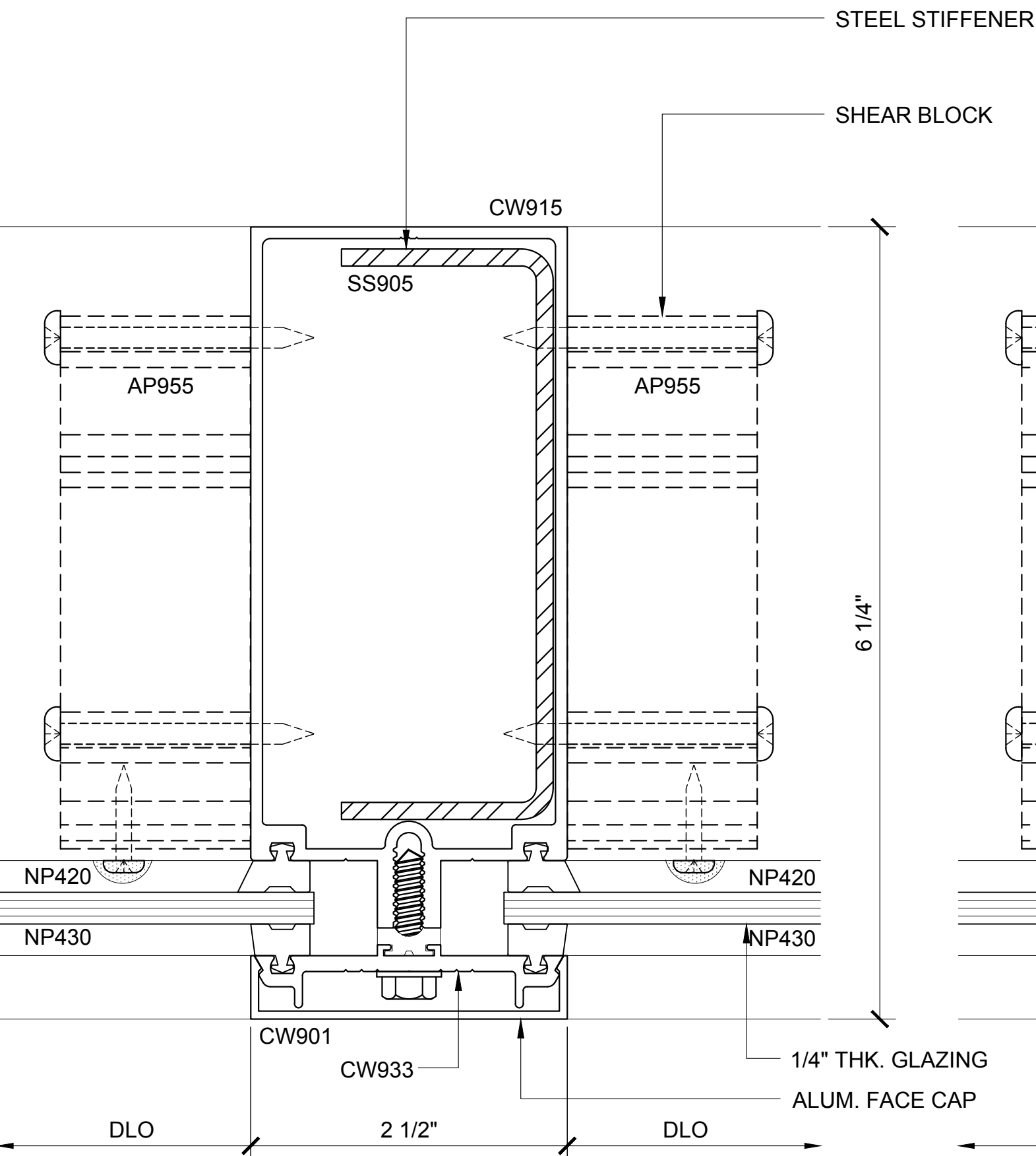
INT. VERT. PLAN 4
