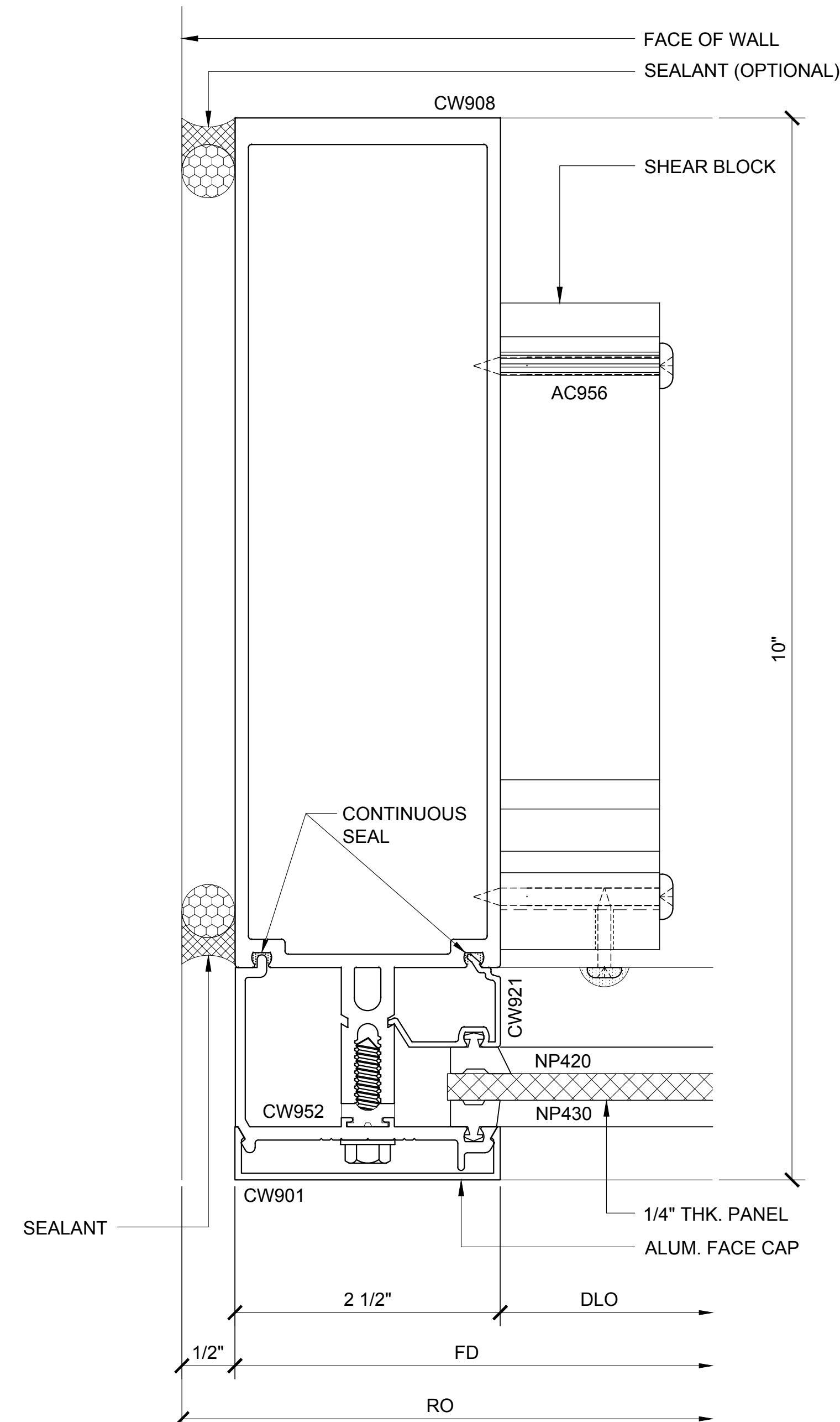
JAMB PLAN 123A
