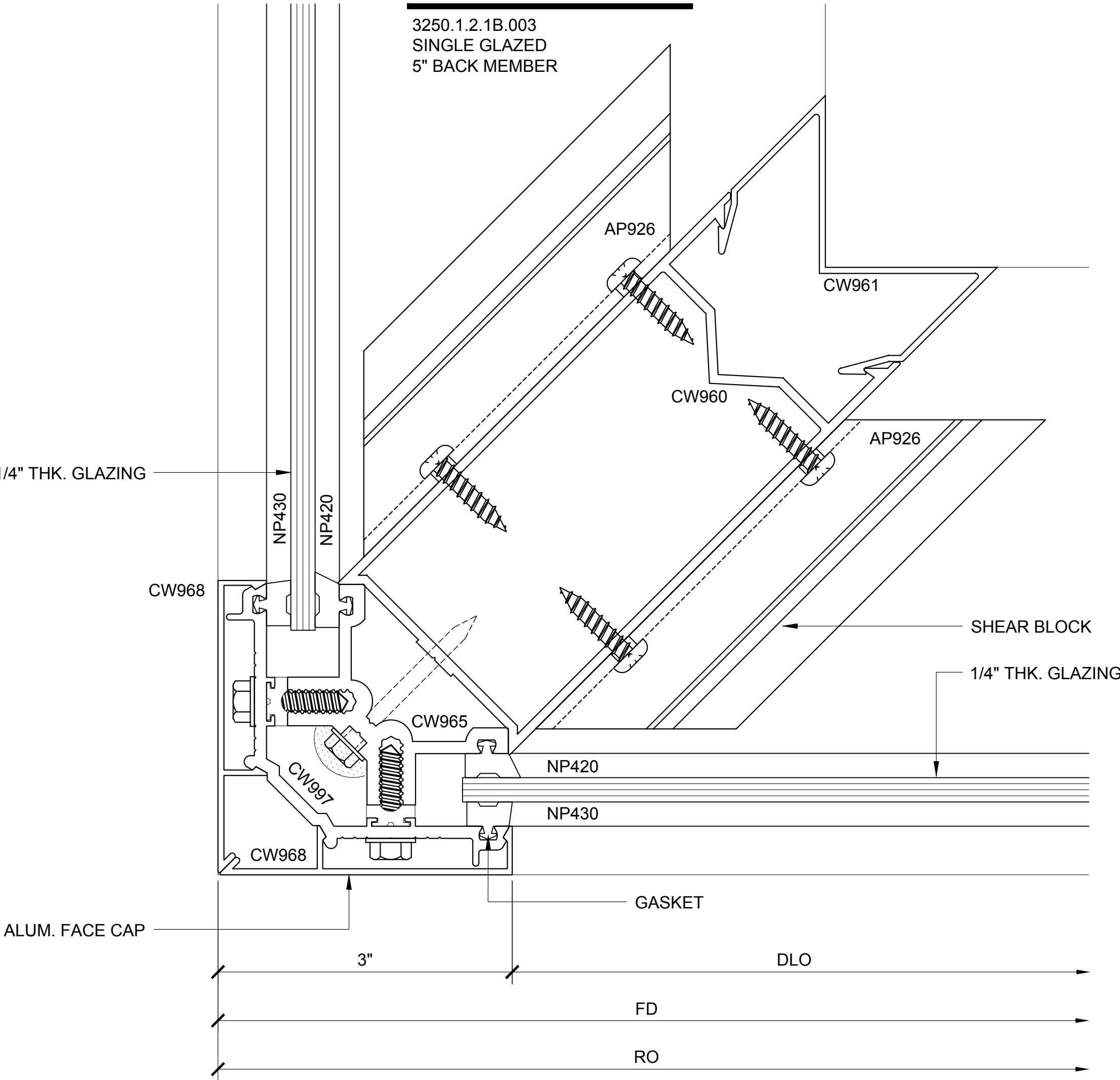
JAMB PLAN 3
