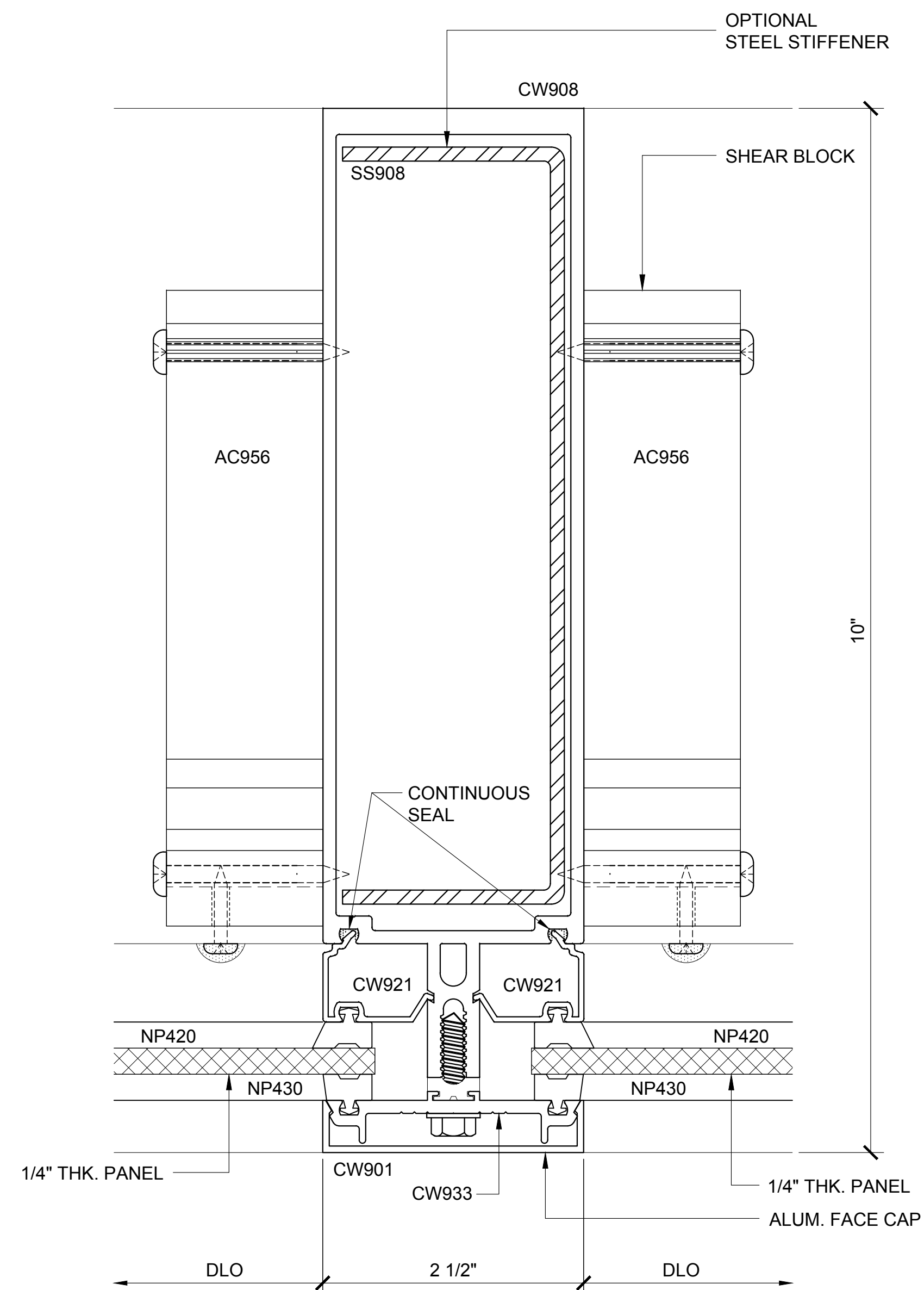
INT. VERT. PLAN 136
