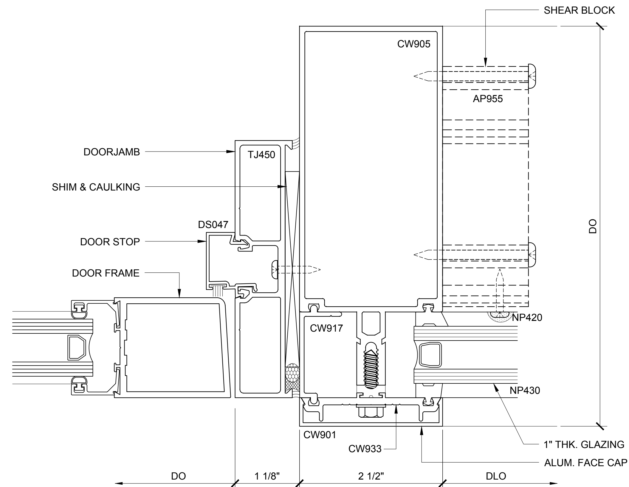
DOOR JAMB PLAN 94
