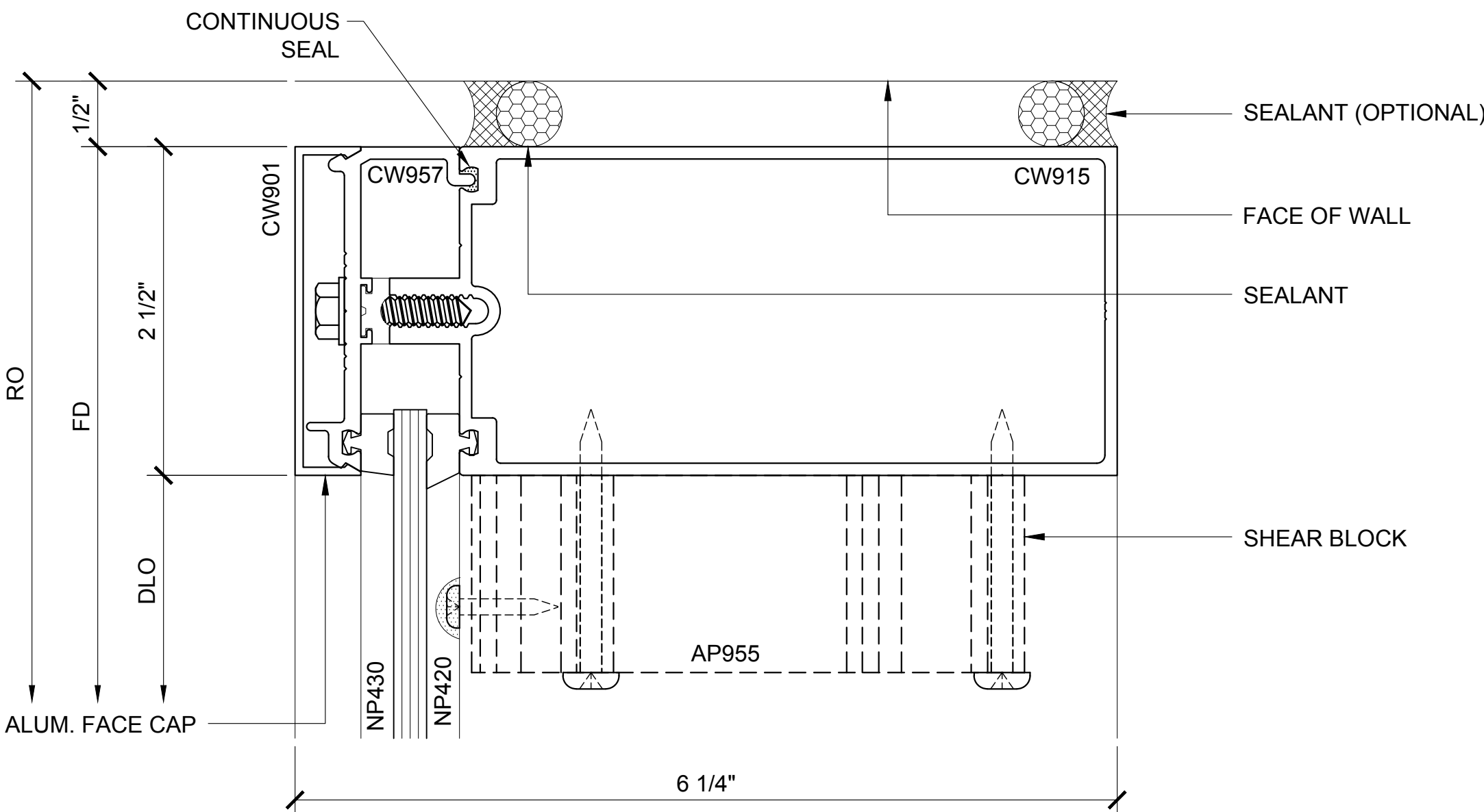
JAMB PLAN 3
