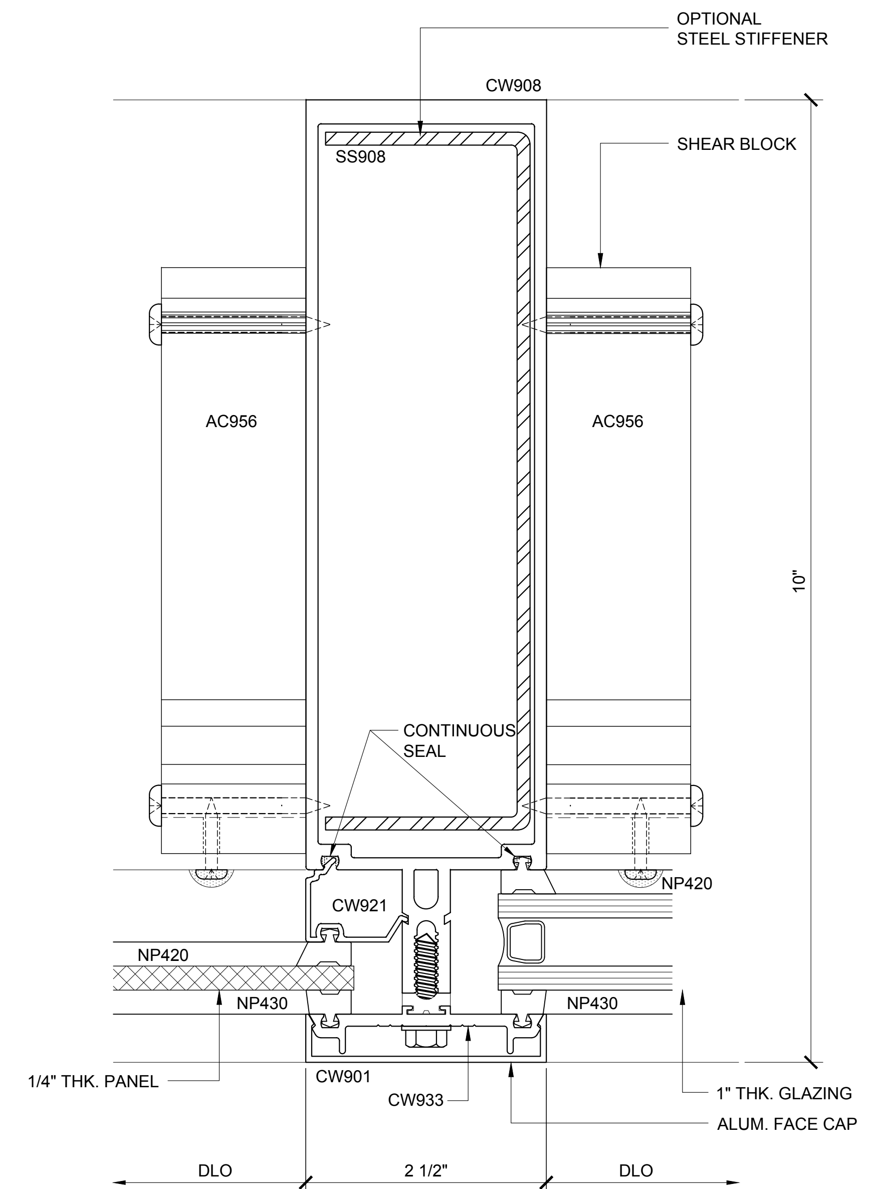
INT. VERT. PLAN 137
