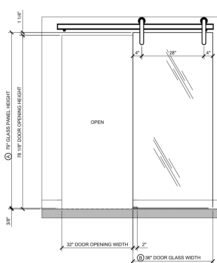
2B ELEVATION
