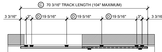
2A PLAN
