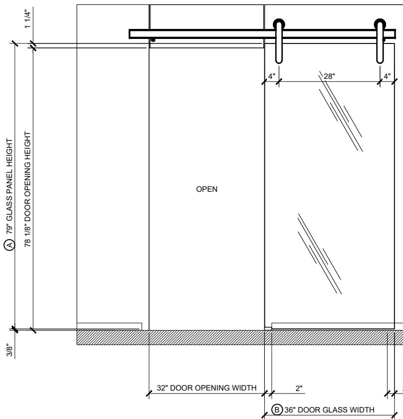
2B ELEVATION
