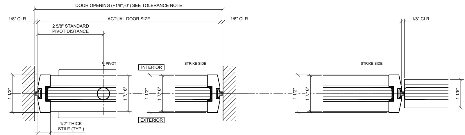
2A PLAN: WALL TO DOOR 2B PLAN: DOOR TO WALL 2C PLAN: DOOR TO SIDELITE
