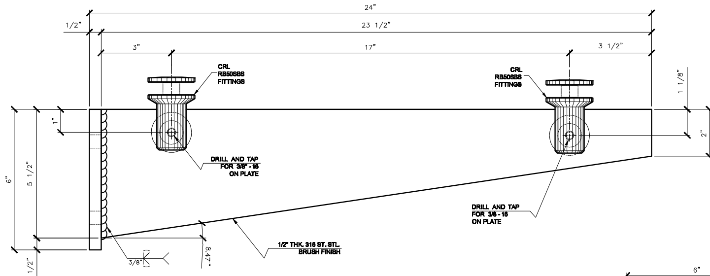
CRL 24" - GAB24 Scale: 1 = 4
