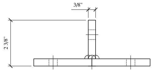
1 AW90VMBS Scale: 1:2
