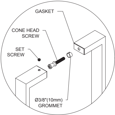
DETAIL A-A
