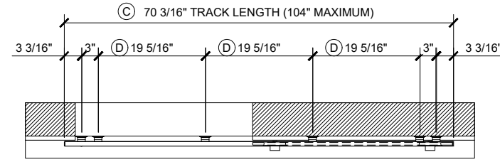
2A PLAN
