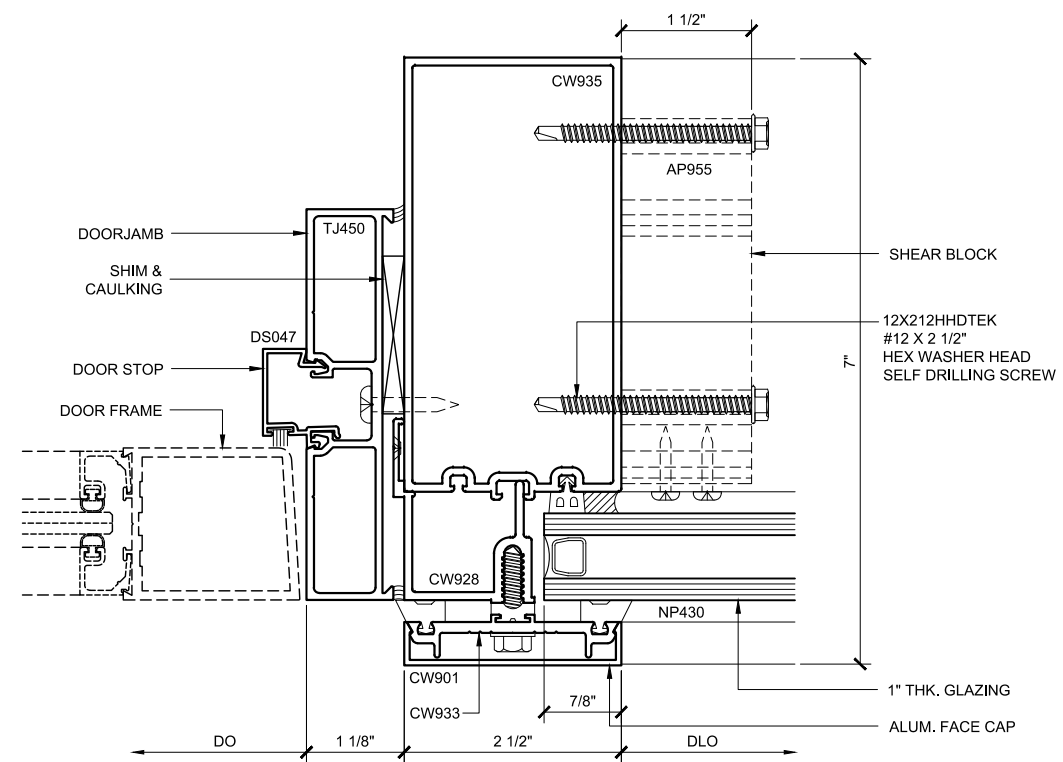
DOOR JAMB PLAN 90
