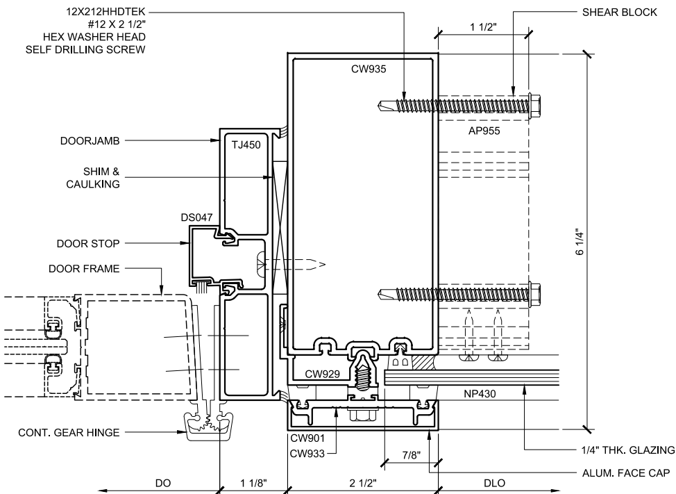
DOOR JAMB PLAN 39
