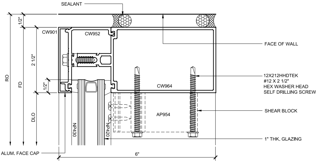
JAMB PLAN 47
