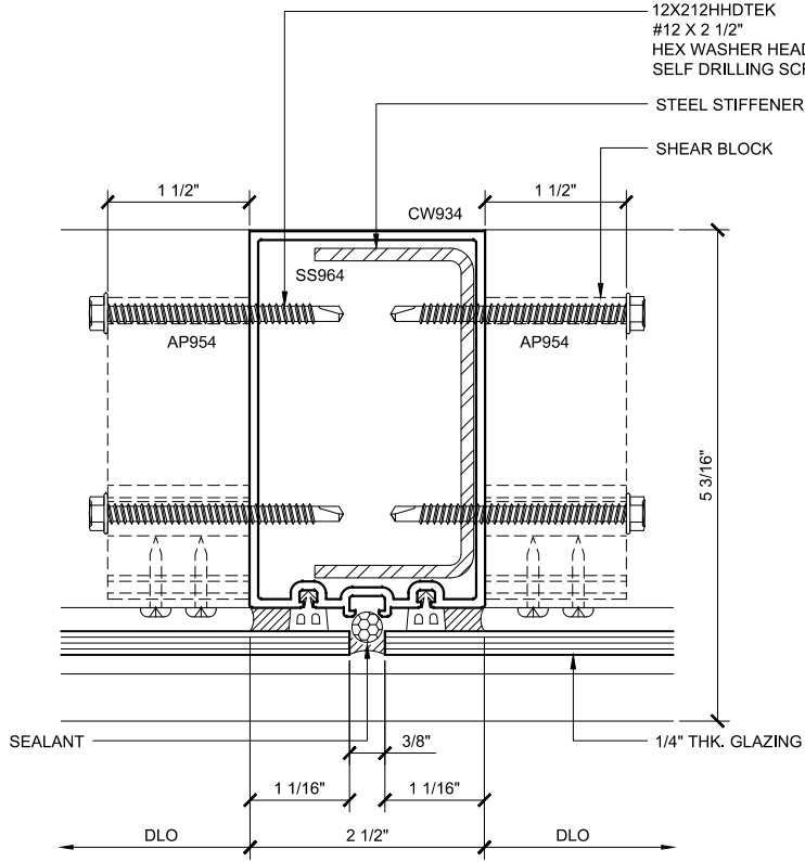
INT. VERT. PLAN ②
