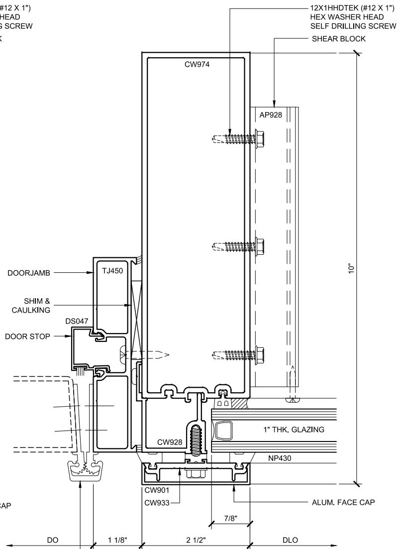
DOOR JAMB PLAN 94
