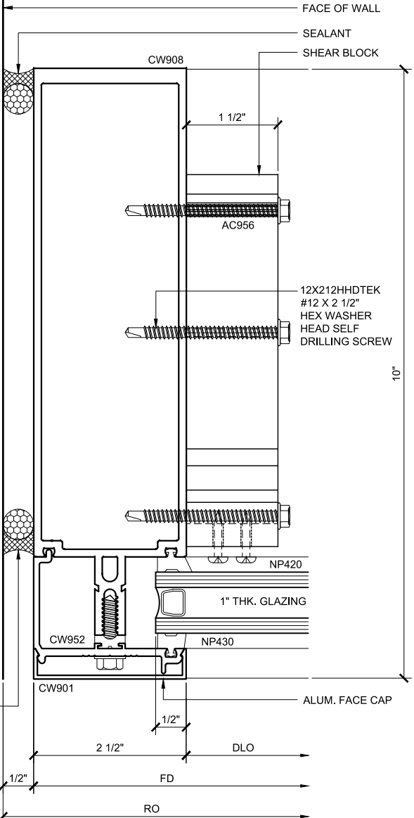
JAMB PLAN 123
