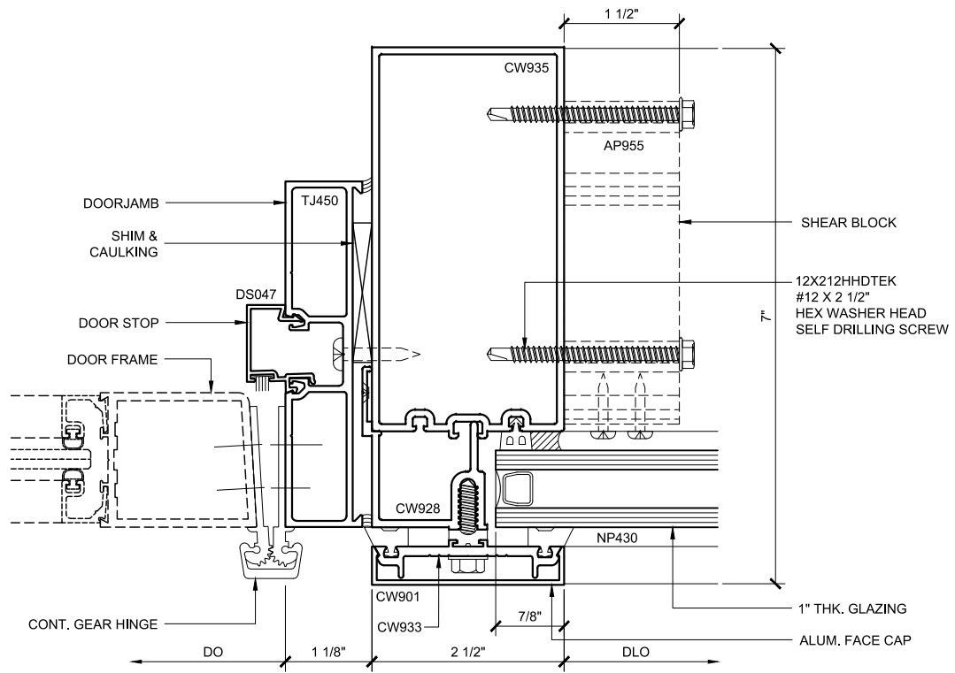
DOOR JAMB PLAN 93
