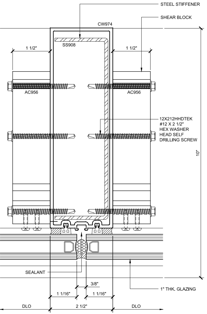
INT. VERT. PLAN 124
