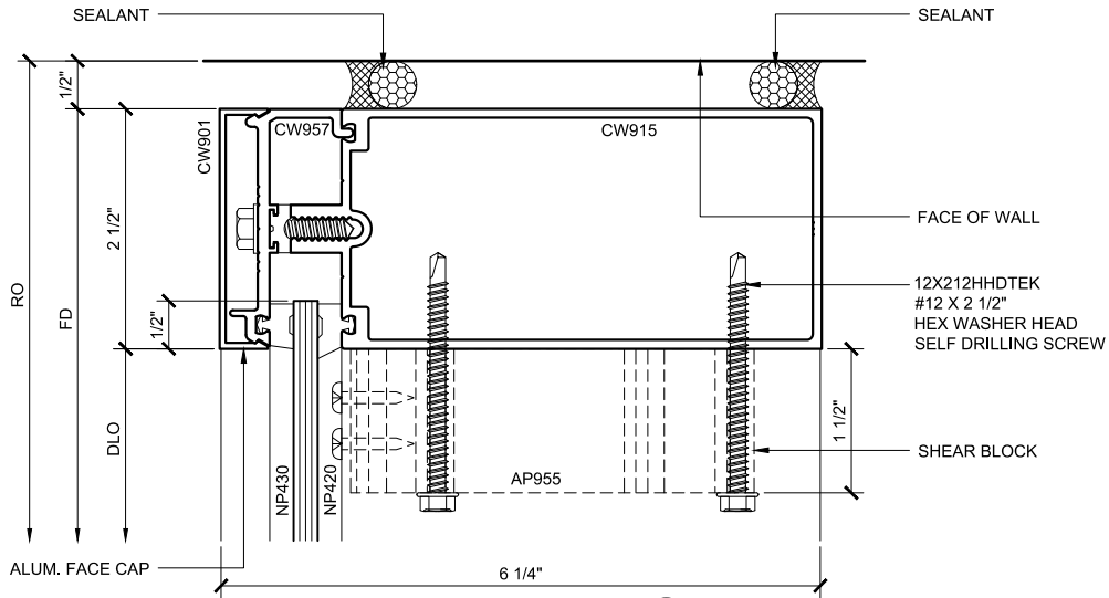
JAMB PLAN 3
