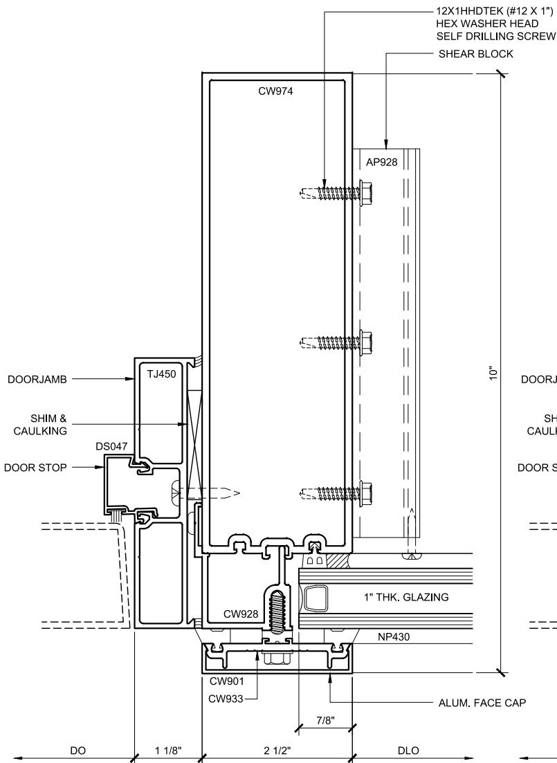
DOOR JAMB PLAN 91
