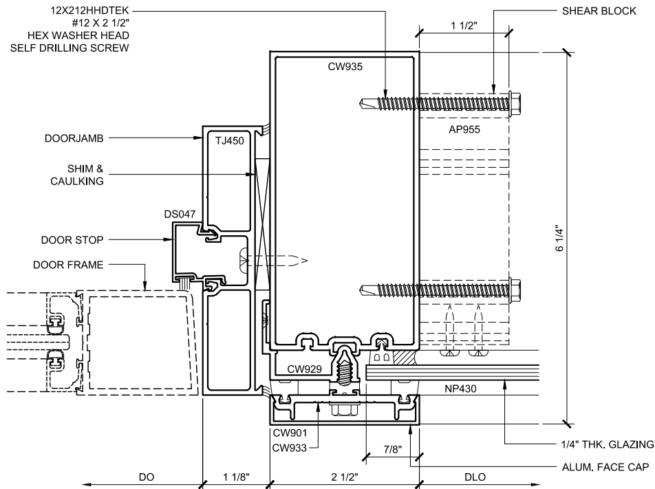
DOOR JAMB PLAN 36
