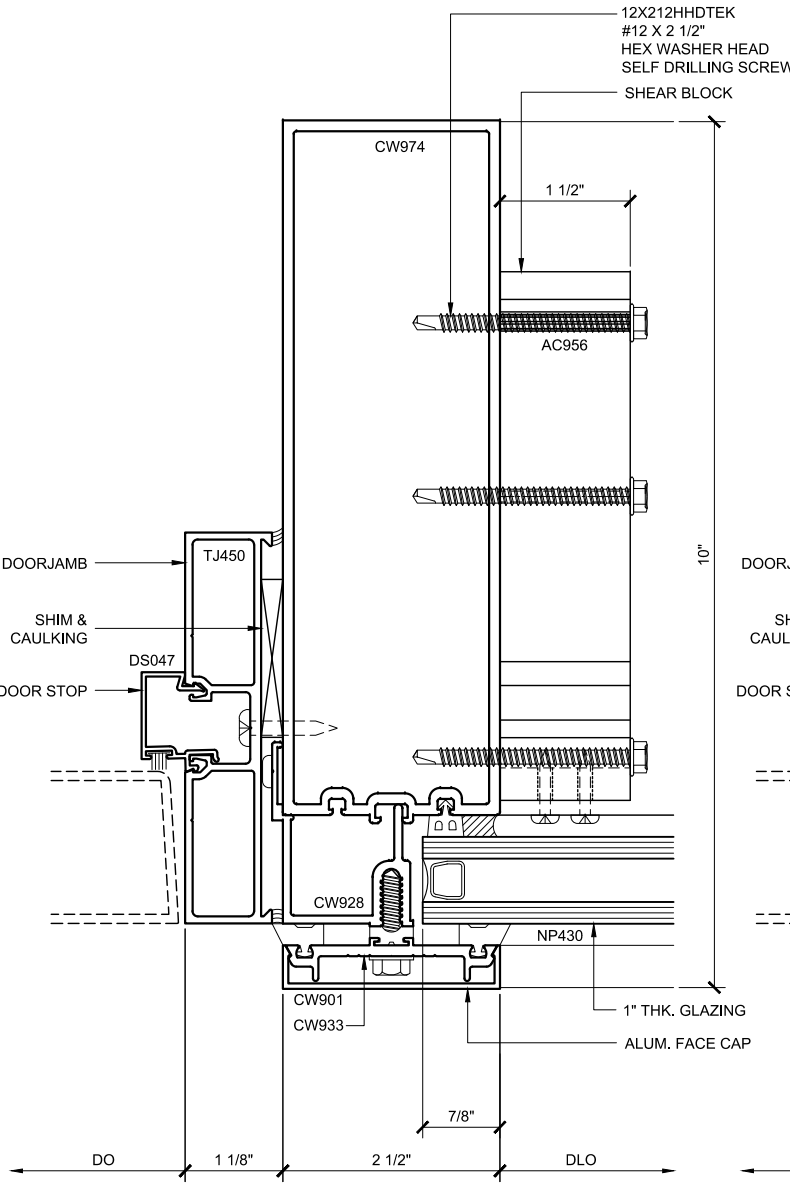
DOOR JAMB PLAN 130
