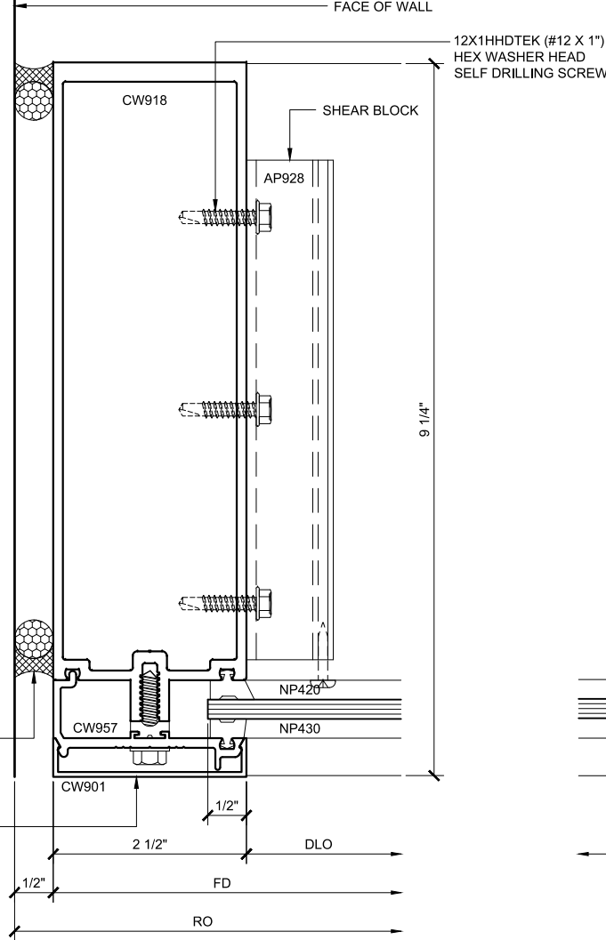
JAMB PLAN 5
