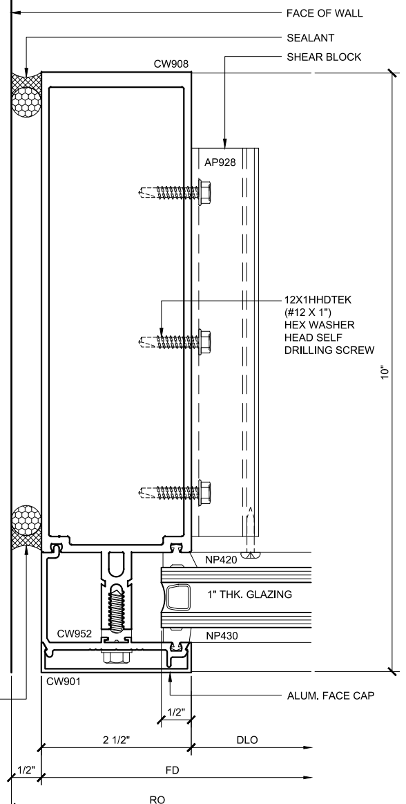
JAMB PLAN 51
