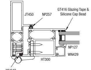
3 HINGE JAMB
