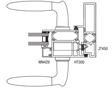
3 HINGE JAMB
