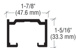
STANDARD D7 OVERHEAD TRACK SPECIFY D1038 ASSEMBLY
