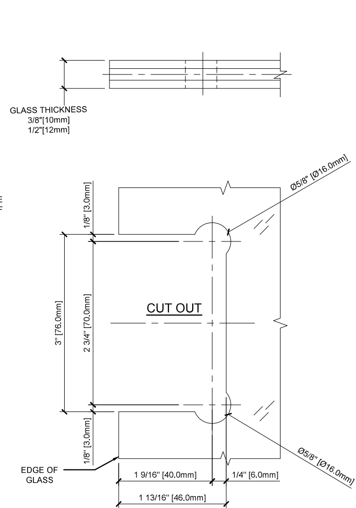
SWING DOOR GLASS TEMPLATE
