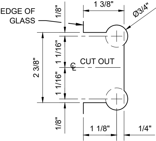
GLASS FABRICATION DOOR TEMPLATE
