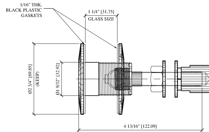
HS1GF14 Scale: 1:1
