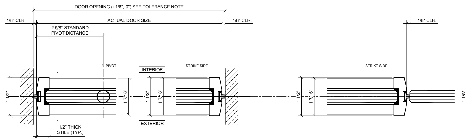
2A PLAN: WALL TO DOOR
